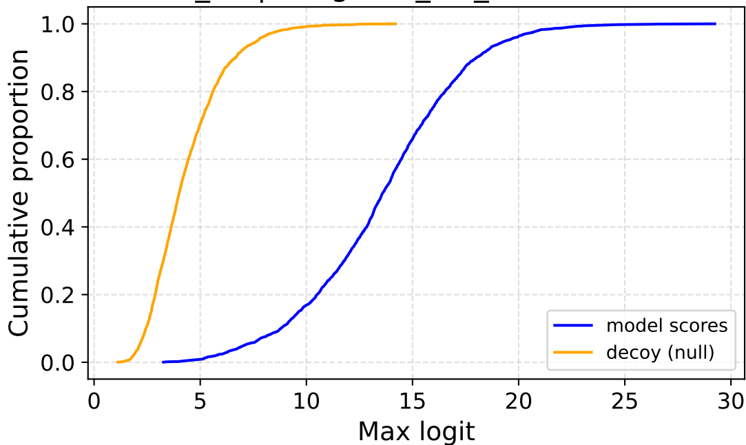
flows_24 | imagenet_val_source — ECDF
