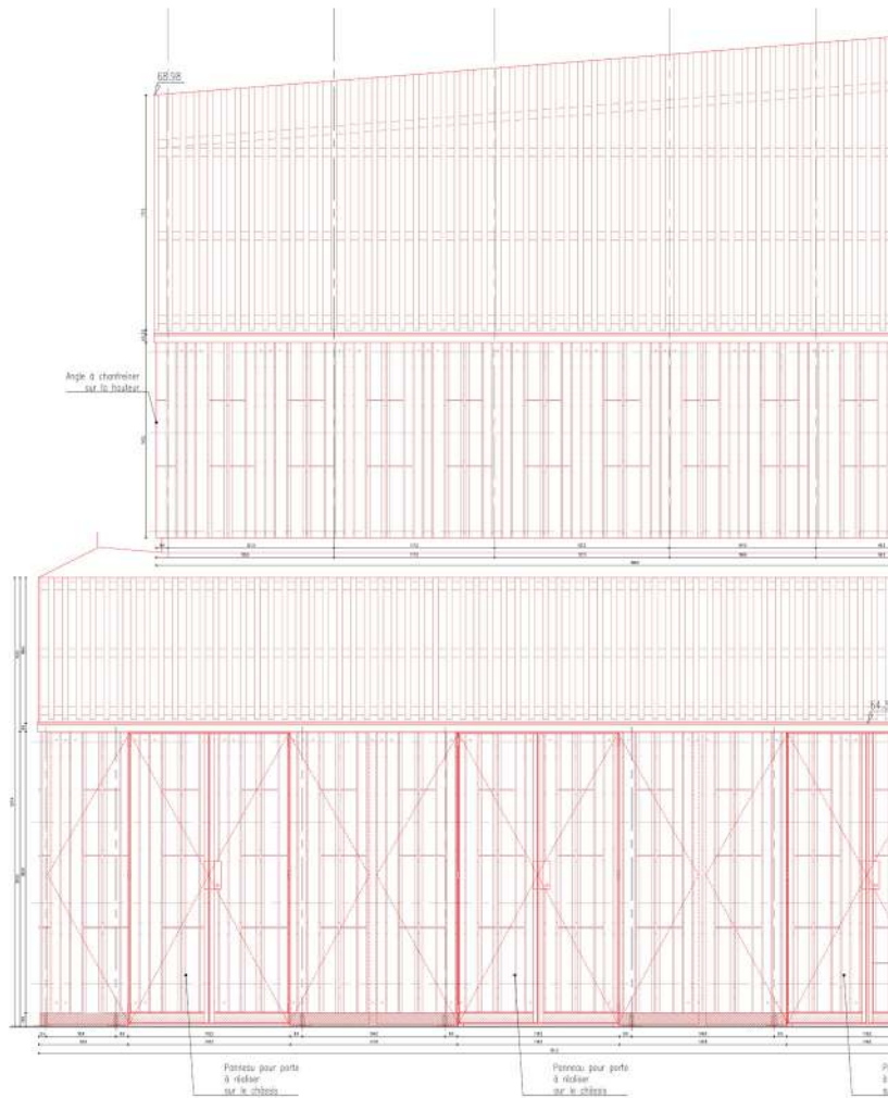
Façade sud-ouest
