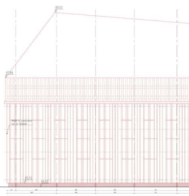
Façade nord-est
