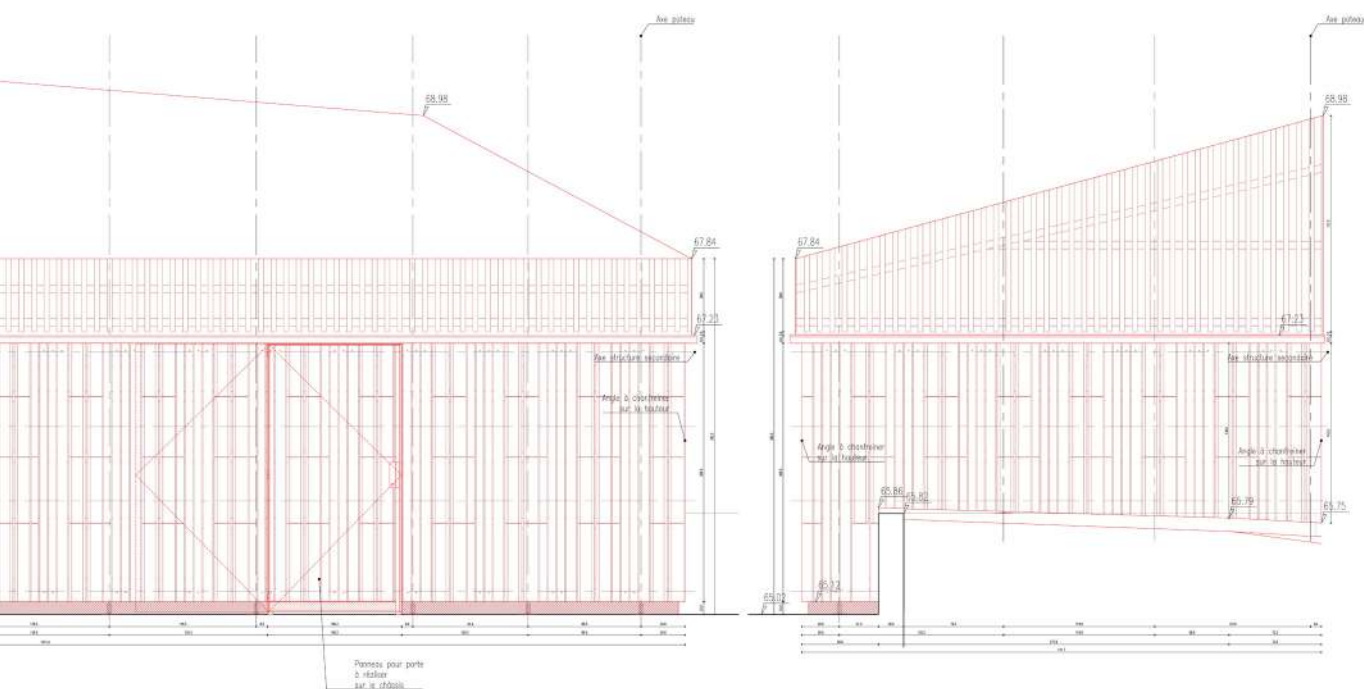
Façade ouest
