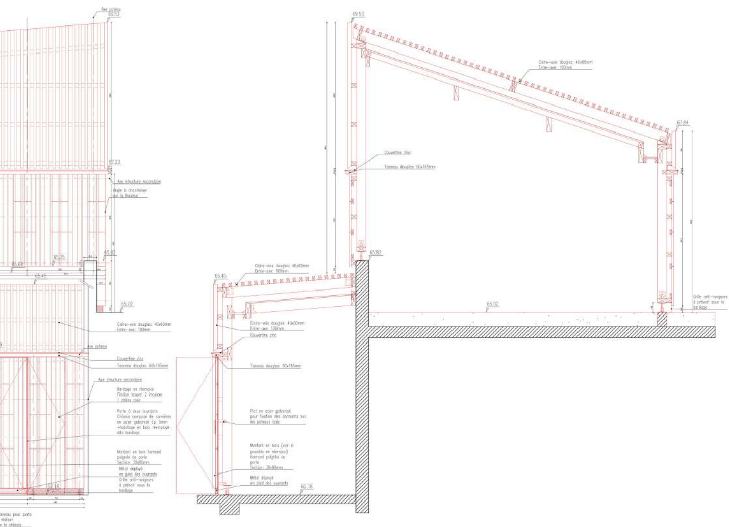
Coupe
