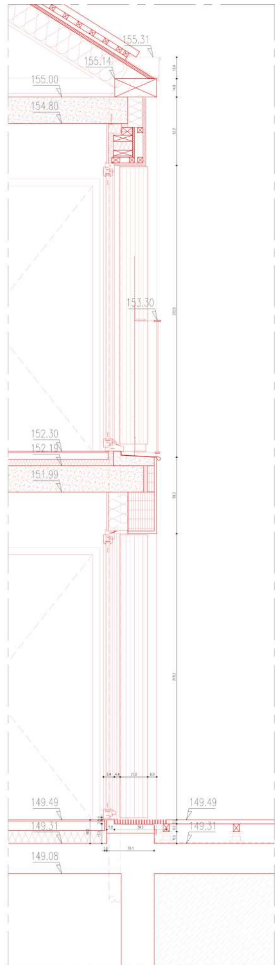
Coupes de détail d'enveloppe.
