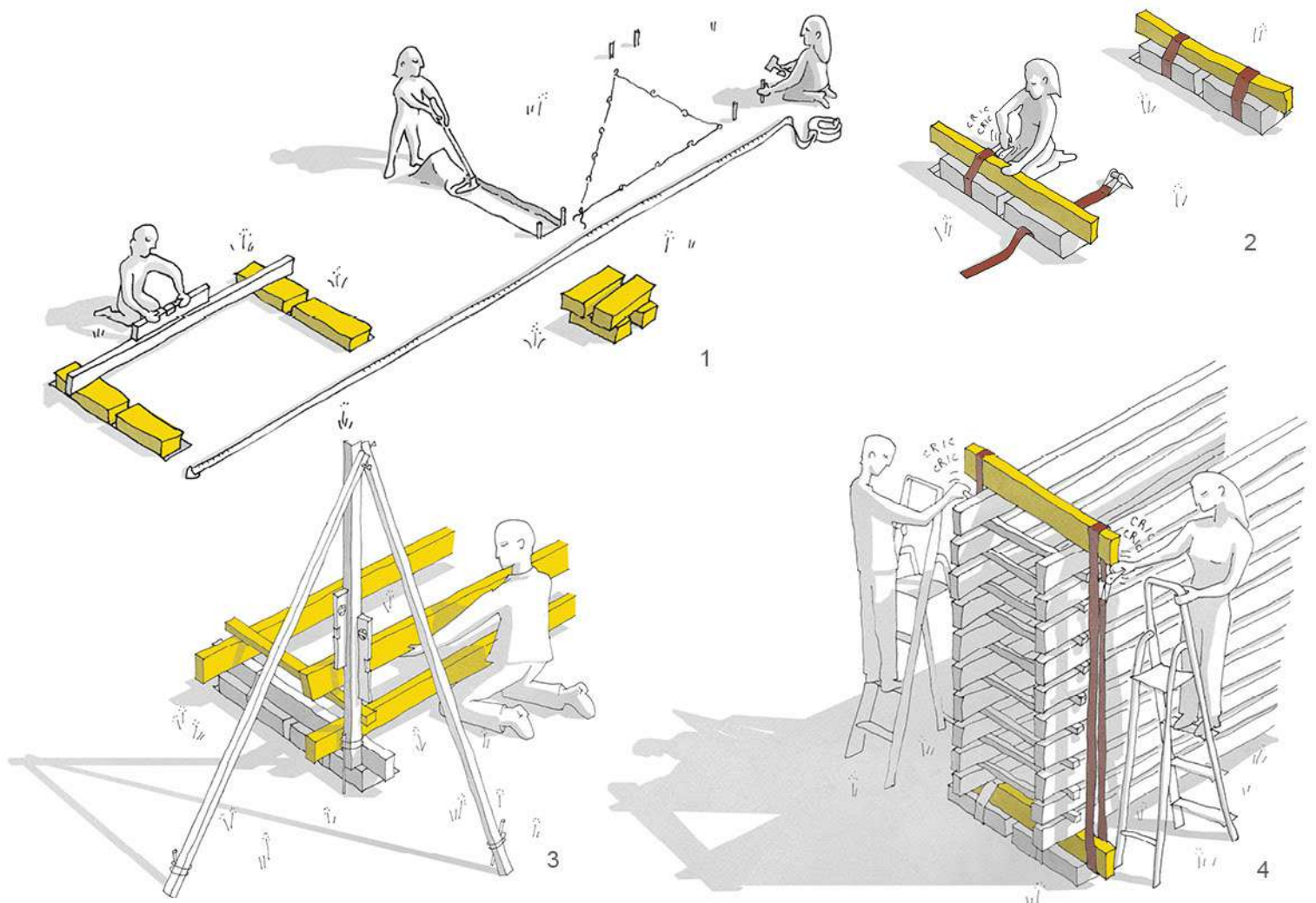
Montage de la cabane.
