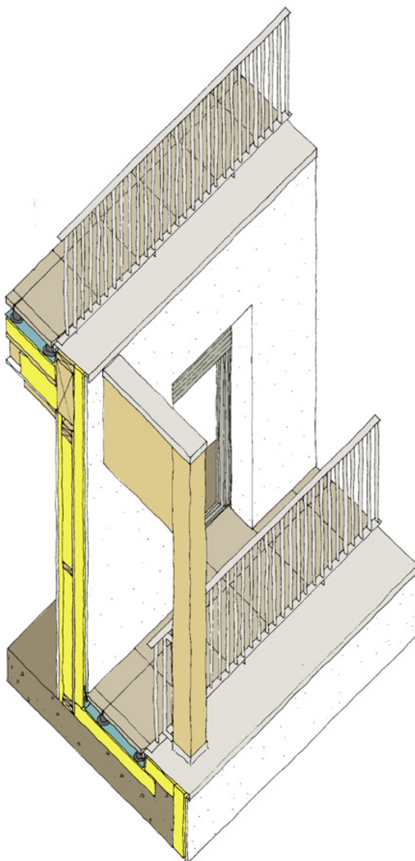
Axonométrie pour la proposition d'un témoin de façade dans le cadre de la réhabilitation d'un ensemble situé rue de la Jonquière à Paris. Dessin réalisé au sein de l'agence d'architecture de Jean Marin et associé-e-s.
