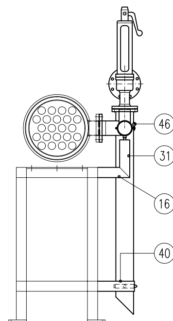
SEZ. A-A
