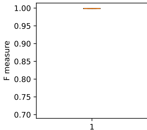
DDoS1 - AdaBoost
