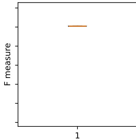
DDoS1 - MLP
