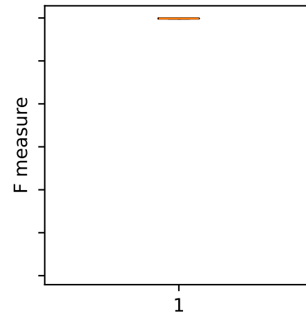
DDoS1 - ID3
