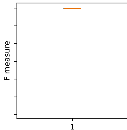
DDoS1 - MLP
