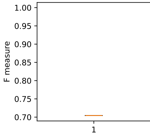
DDoS1 - AdaBoost
