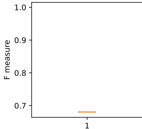
FTP-Patator - AdaBoost
