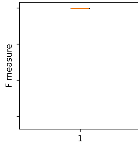
FTP-Patator - ID3
