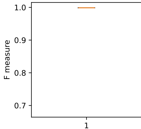
FTP-Patator - AdaBoost
