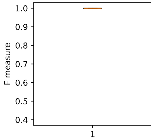
Heartbleed - AdaBoost
