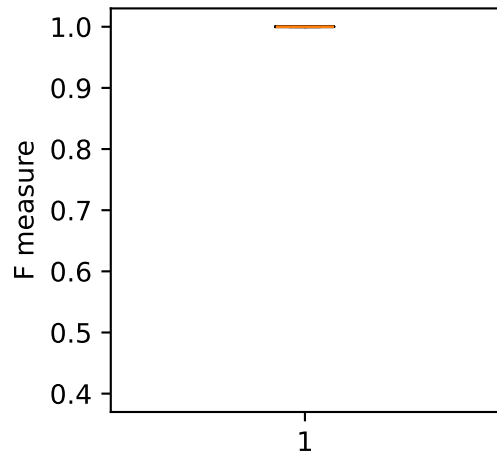
Heartbleed - AdaBoost
