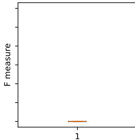
Heartbleed - MLP
