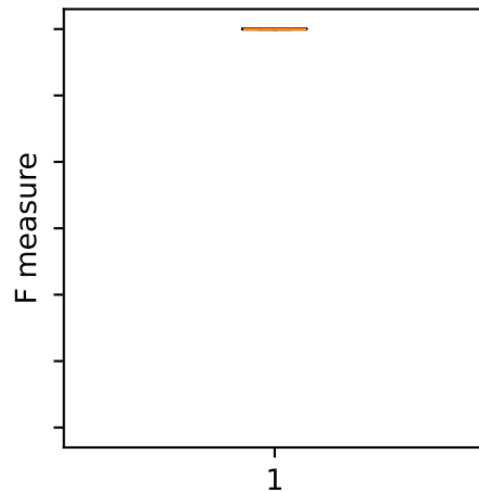
Heartbleed - MLP
