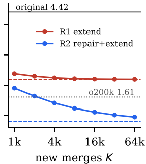
Qwen3
