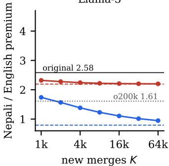
Llama-3
