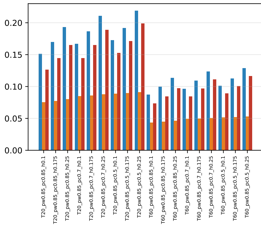
Mean CI width
