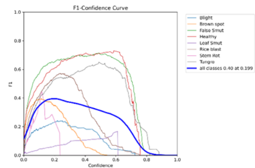
Fig. 12. F1 Curve
