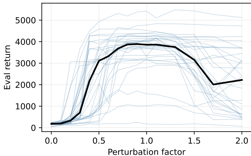
KL \rho = 0.05
