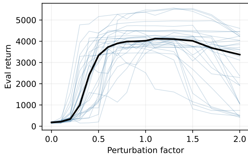
KL \rho = 0
