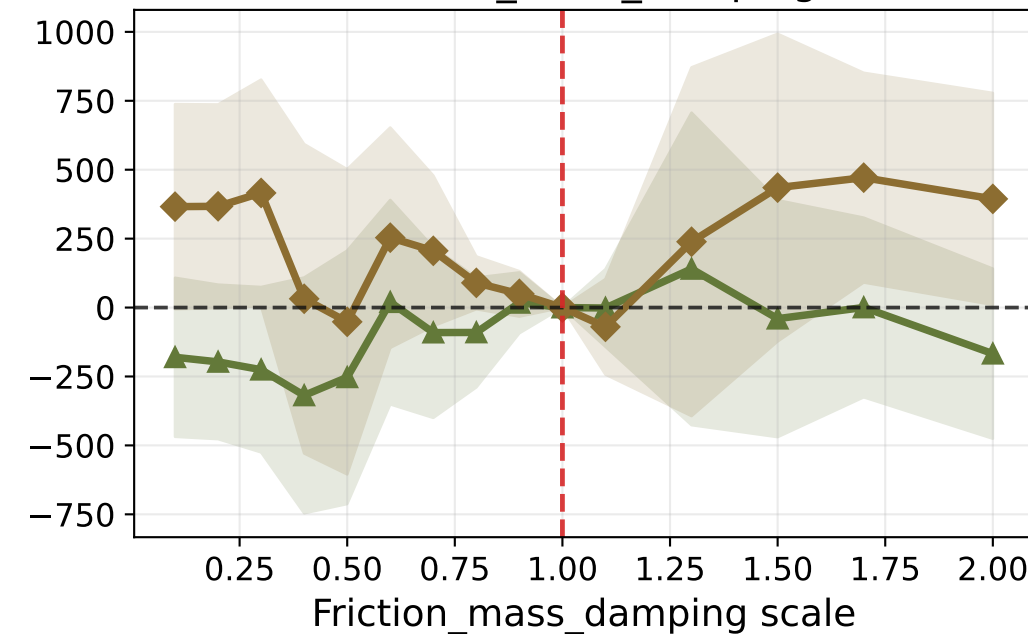
Friction_mass_damping
