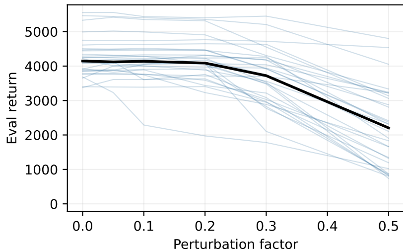
KL \rho = 0
