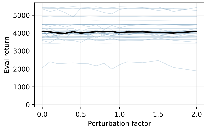
KL \rho = 0
