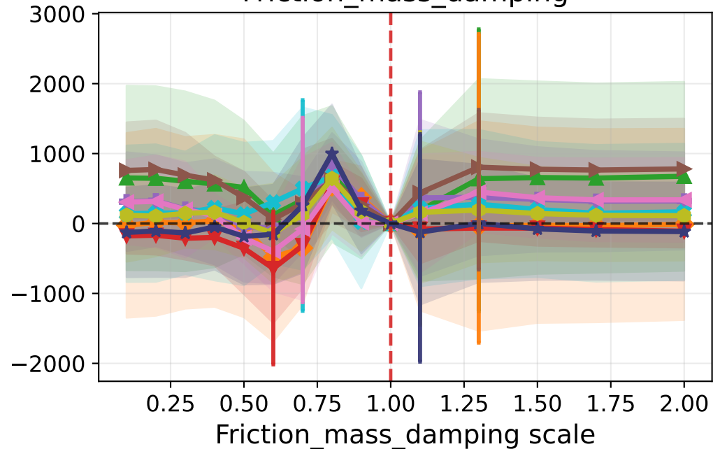
Friction_mass_damping
