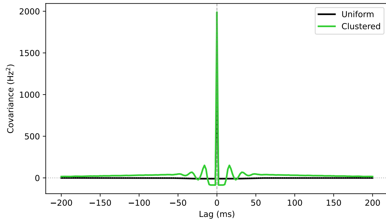
Autocovariance
