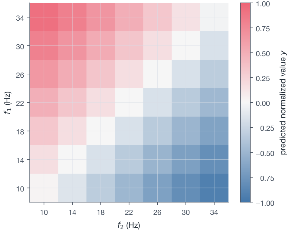
Predicted y | MSE=3.73e-04
