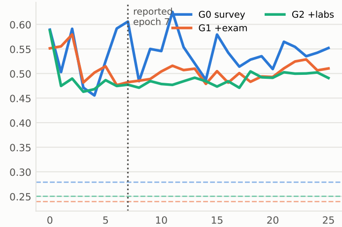
NHANES · \gamma 0.5, per-step
