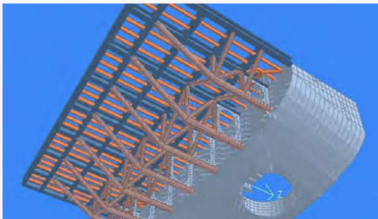
DESIGN AND FABRICATION OF A CANTILEVER. DISEÑO Y FABRICACIÓN DE AMPLIACIÓN DE CUBIERTA.
