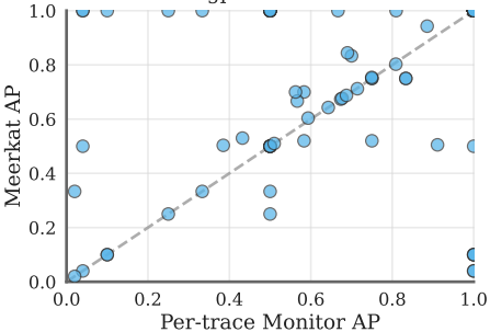
gpt-5.4-mini
