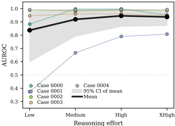
Per-case AUROC trajectories
