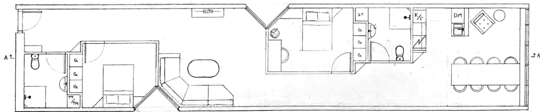
PLAN 1:50
