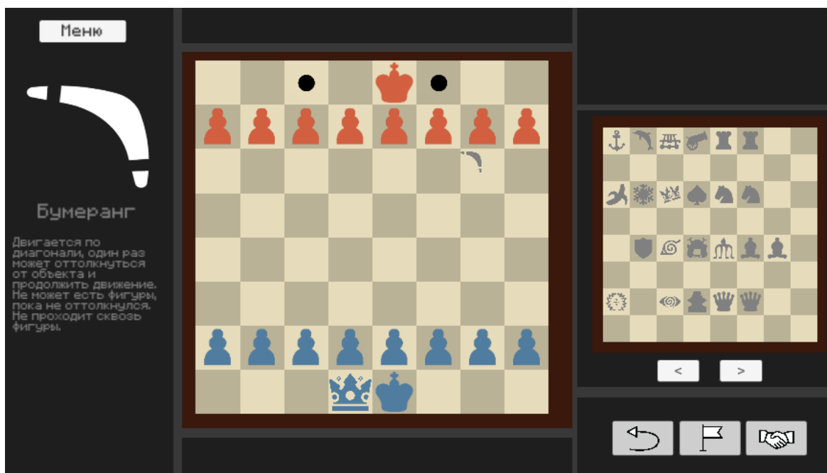
Рисунок 4 Драфт
