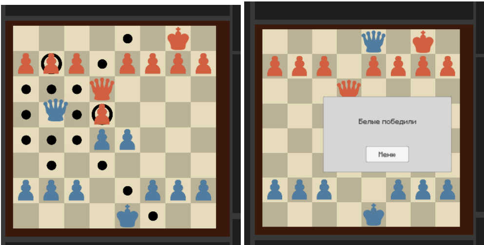
Рисунок 6 Ситуация мата
