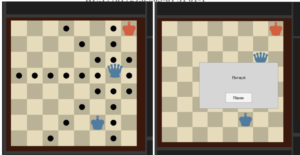
Рисунок 7 Ситуация пата
