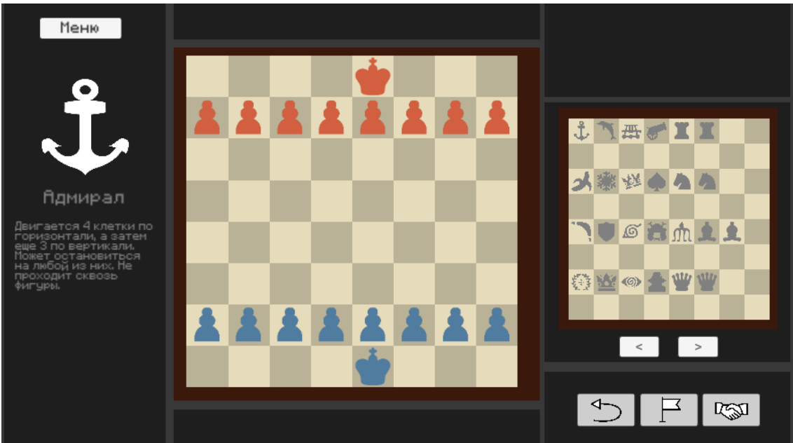
Рисунок 2 Меню матча
