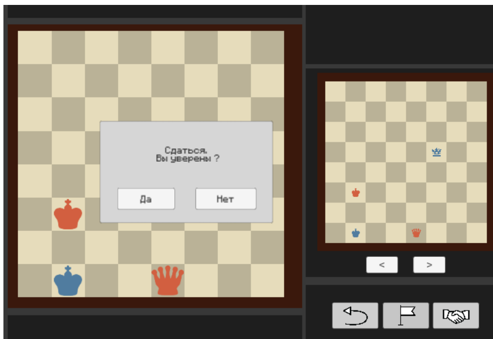
Рисунок 11 Попытка сдаться
