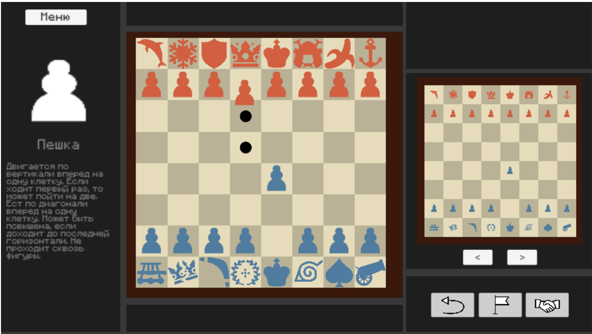
Рисунок 5 Процесс игры
