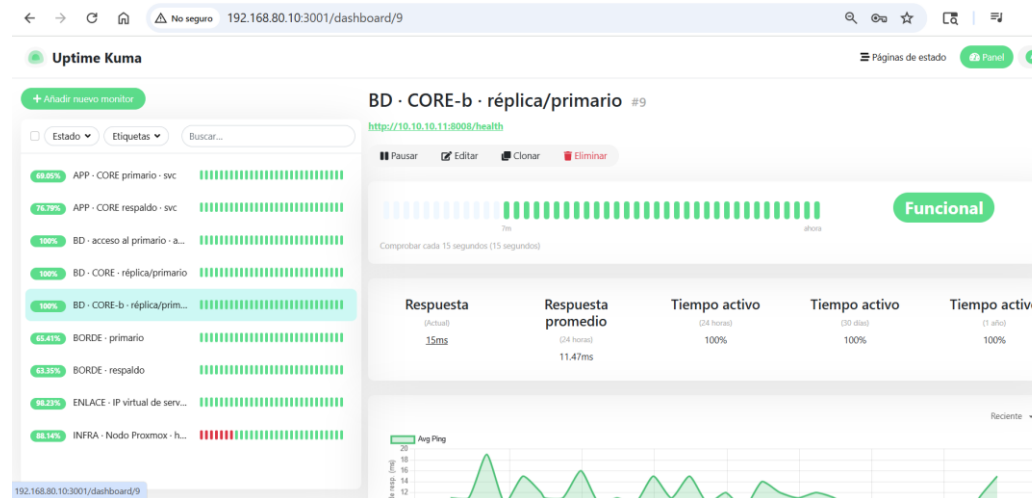
Figura 27. BD · CORE-b · réplica/primario
