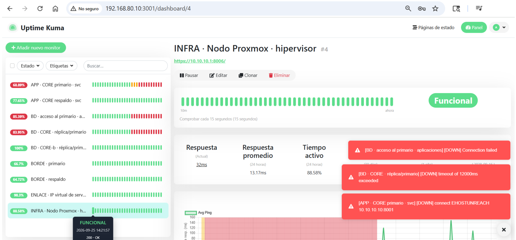
Figura 51. P1: el monitoreo detecta la falla
