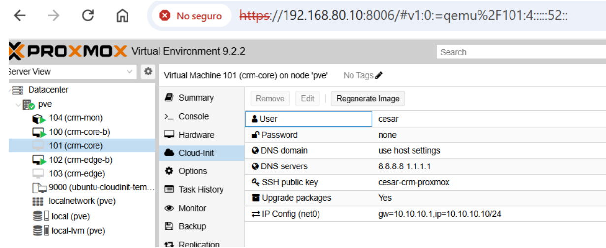
Figura 53. P2: Proxmox con crm-edge apagado
