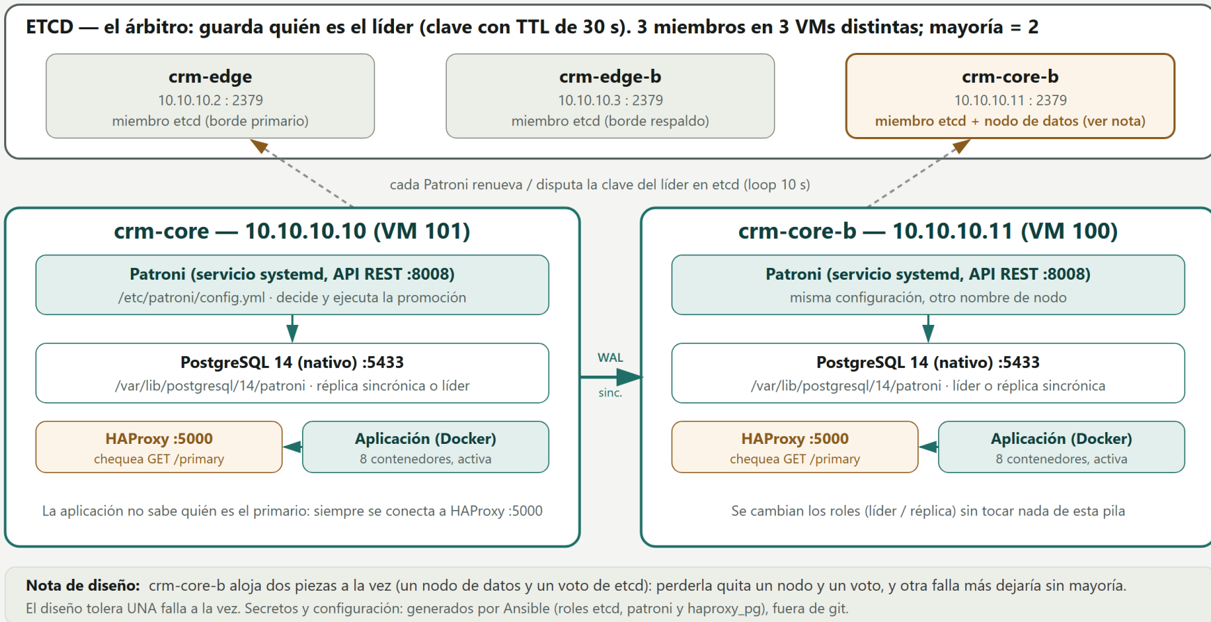
Figura 45. Alta disponibilidad de la base de datos: dónde vive cada pieza
