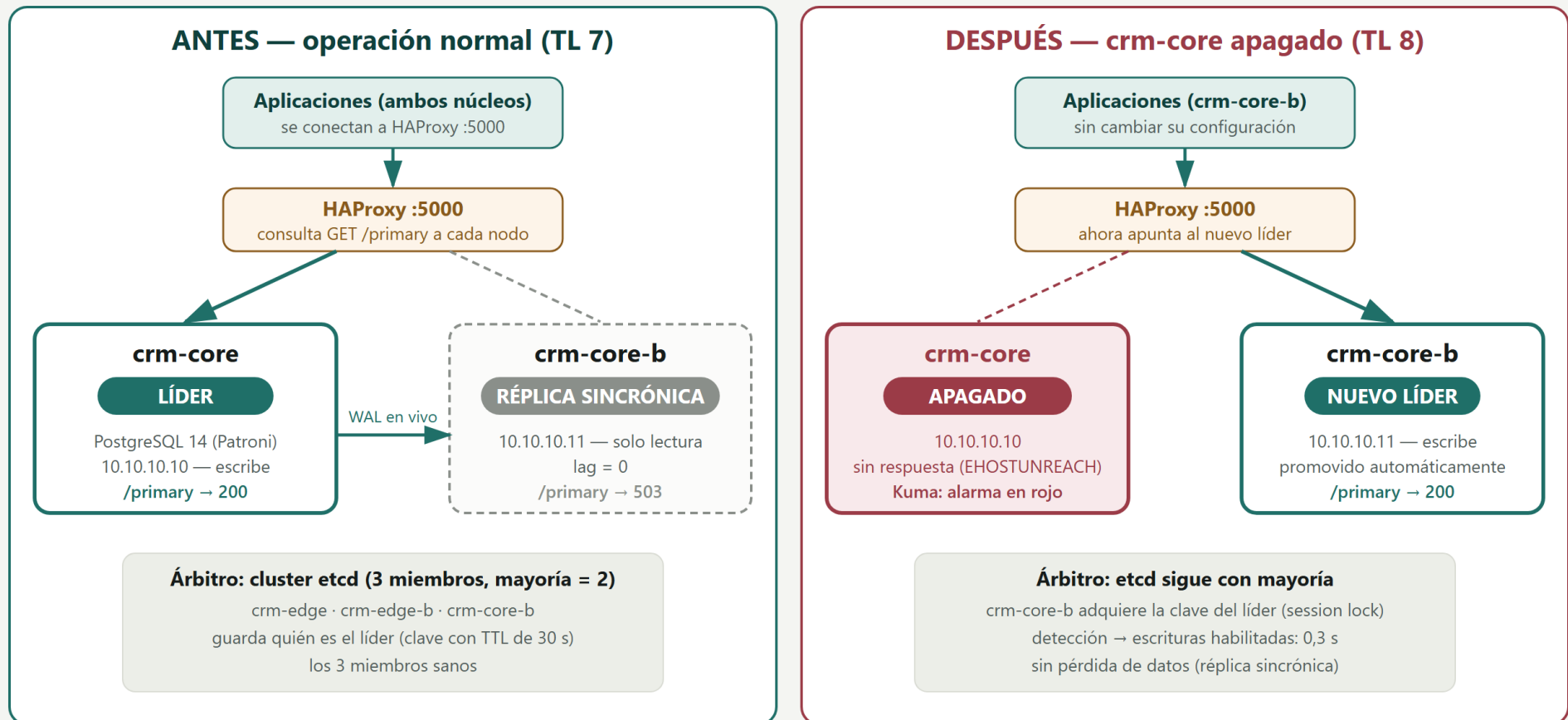
Figura 46. Conmutación automática de la base de datos: antes y después
