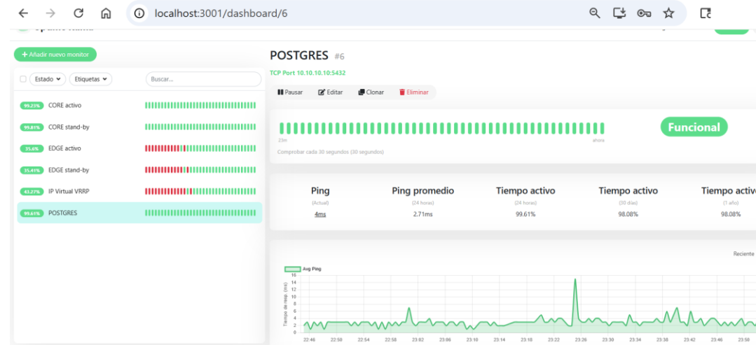
Figura 38. Etapa 1: monitor POSTGRES (TCP 10.10.10.10:5432)
