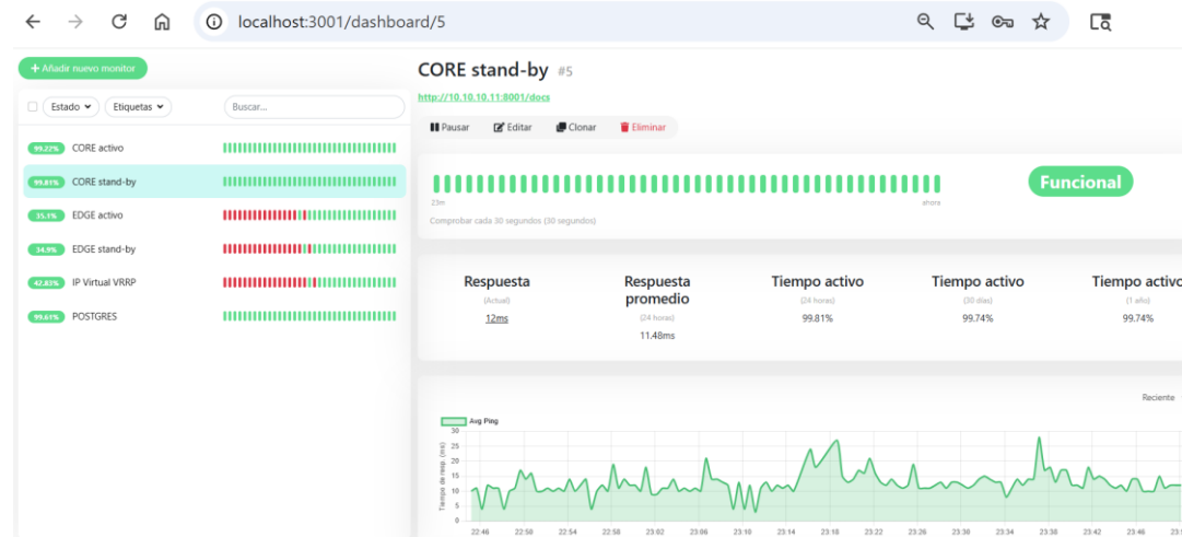
Figura 34. Etapa 1: monitor CORE stand-by (10.10.10.11:8001)
