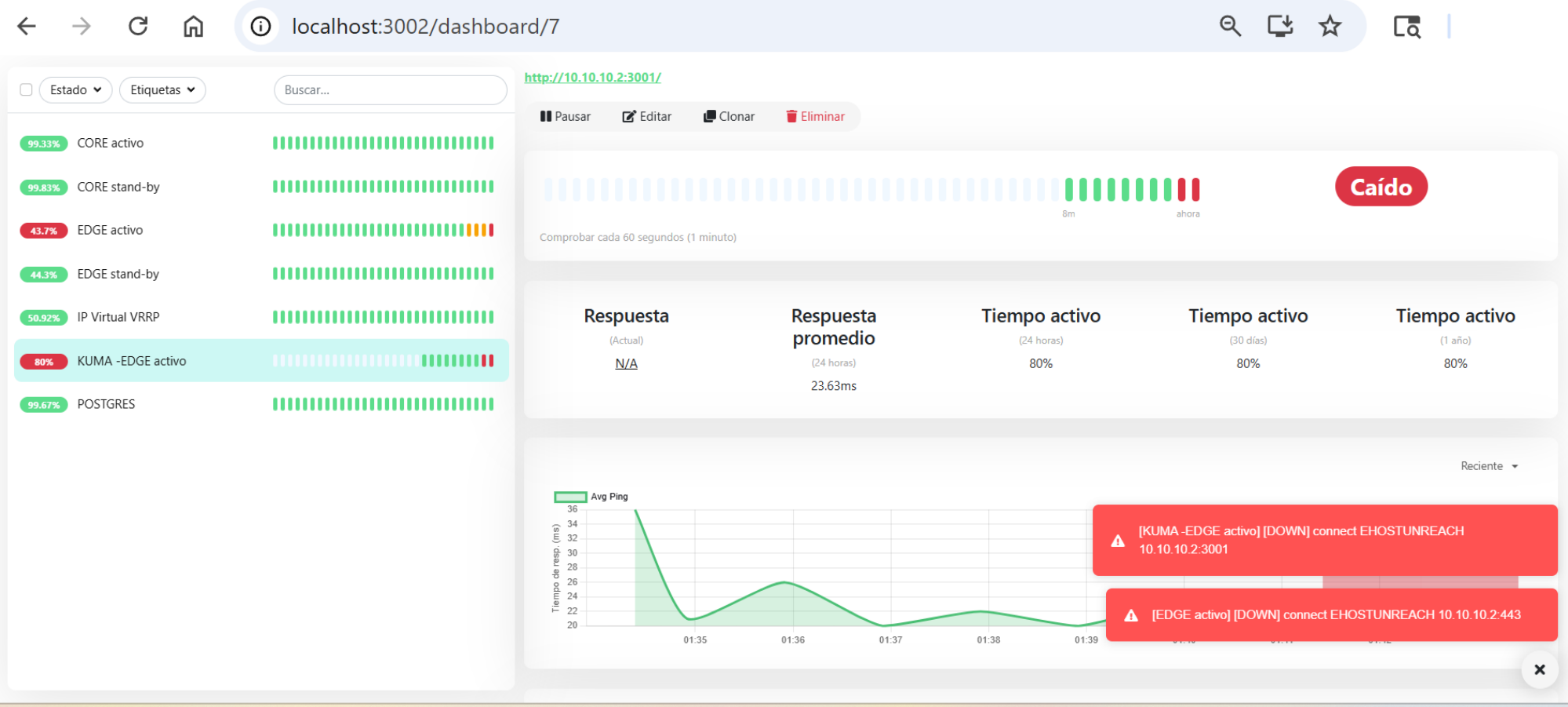
Figura 40. Etapa 2: prueba de estrés con la instancia de crm-edge b
