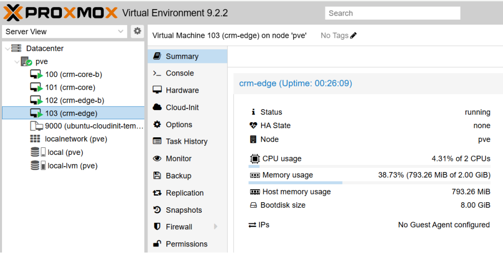
Figura 90. Resumen de crm-edge (VM 103)
