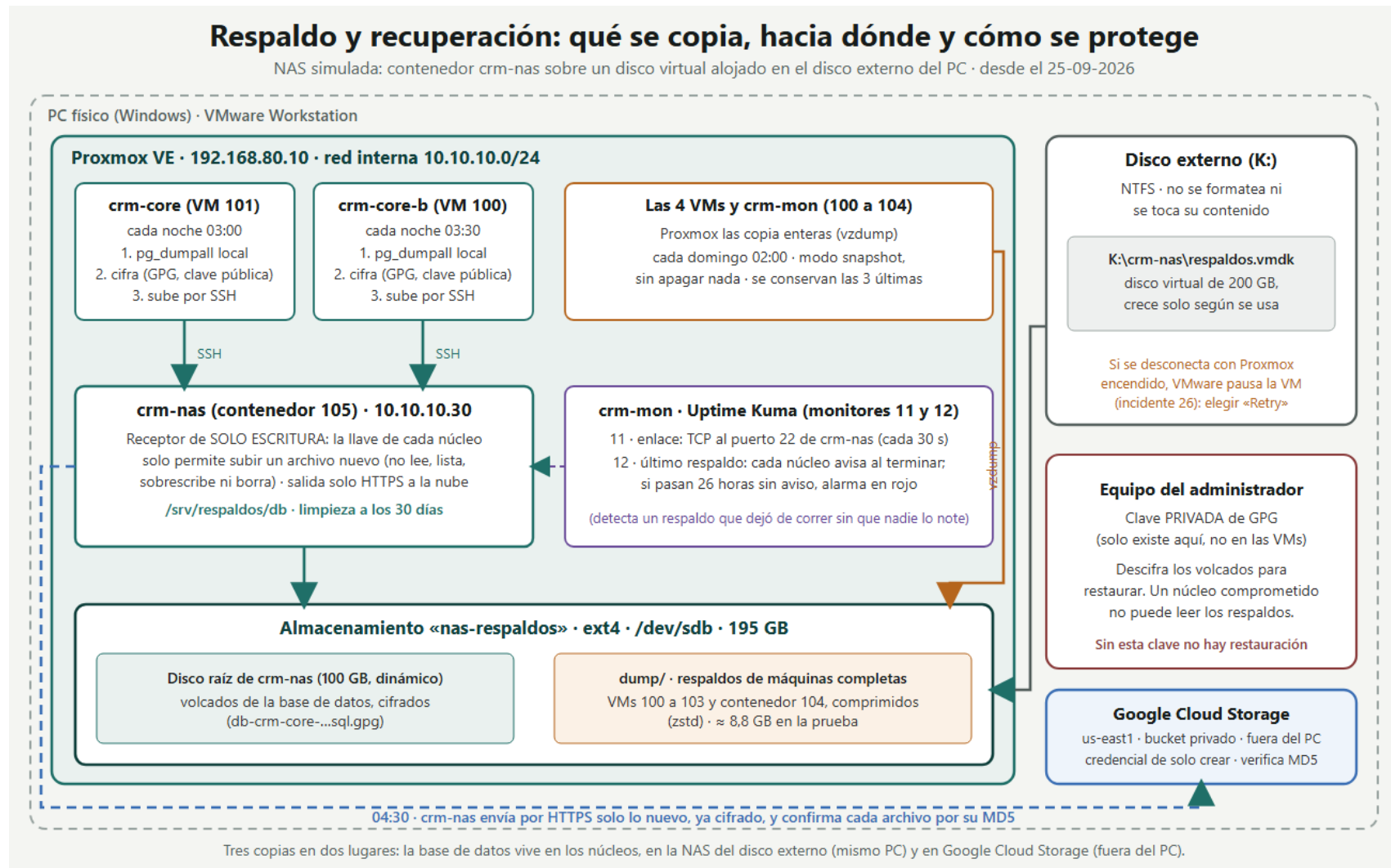
Figura 53. Respaldo y recuperación: qué se copia, hacia dónde y cómo se protege
