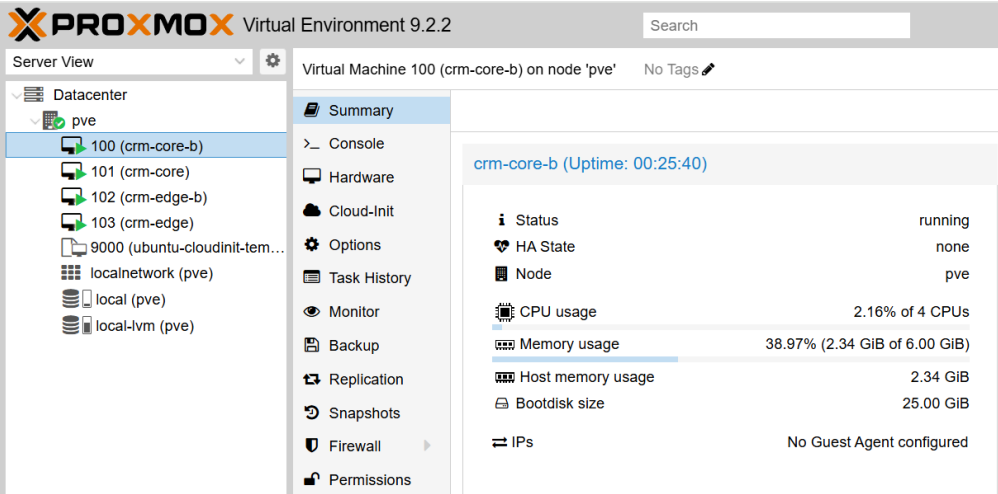
Figura 87. Resumen de crm-core-b (VM 100)
