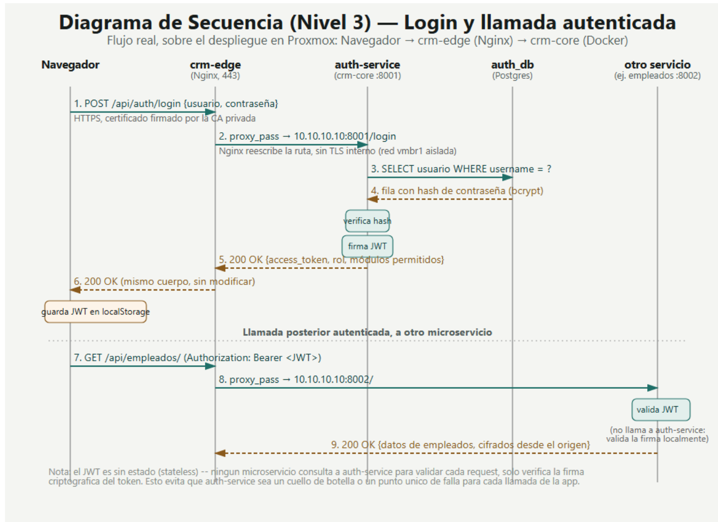
Figura 97. Diagrama de secuencia del inicio de sesión (nivel 3)
