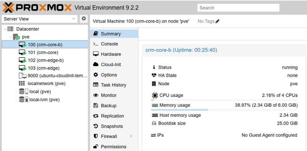
Figura 77. Resumen de crm-core-b (VM 100)
