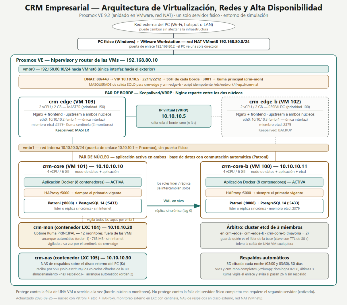
Figura 2. Vista física: infraestructura de virtualización y red
