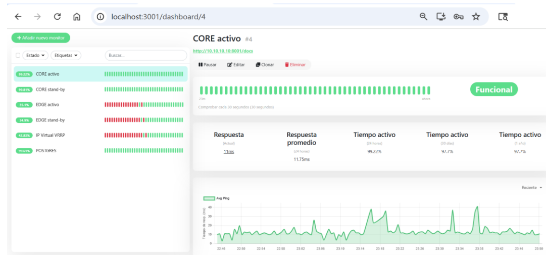
Figura 38. Etapa 1: monitor CORE activo (10.10.10.10:8001)
