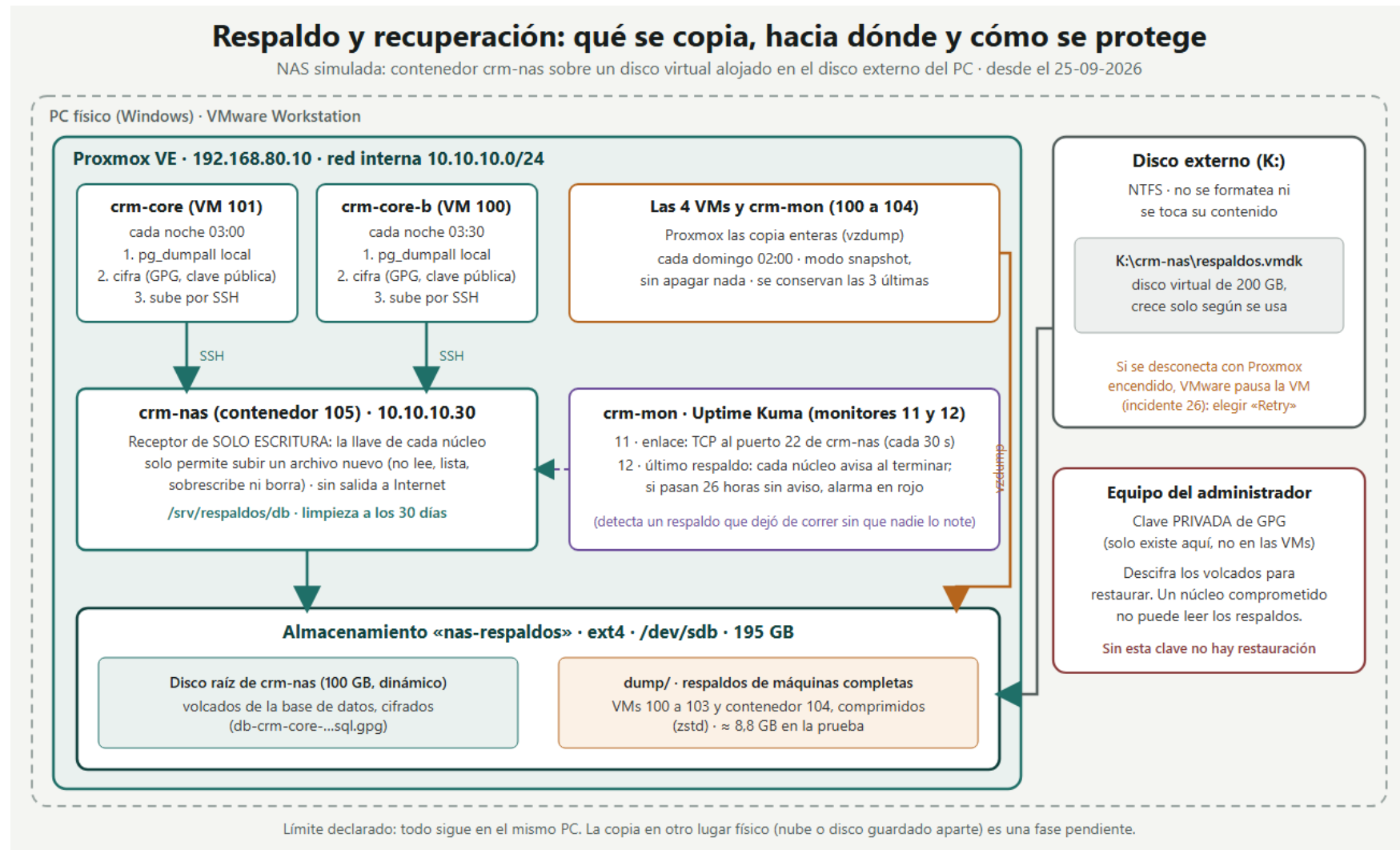
Figura 52. Respaldo y recuperación: qué se copia, hacia dónde y cómo se protege
