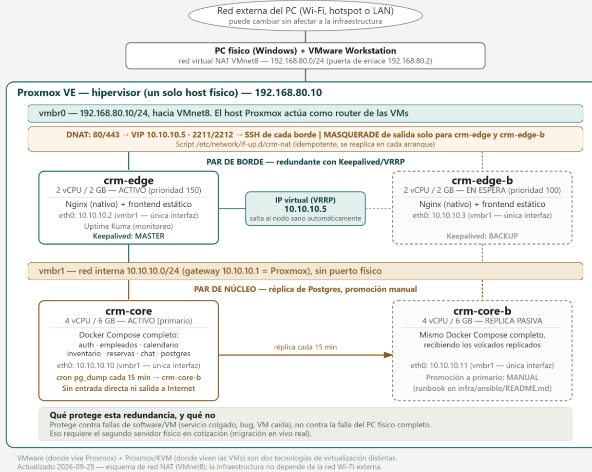
Figura 5. Vista física: infraestructura de virtualización y red
