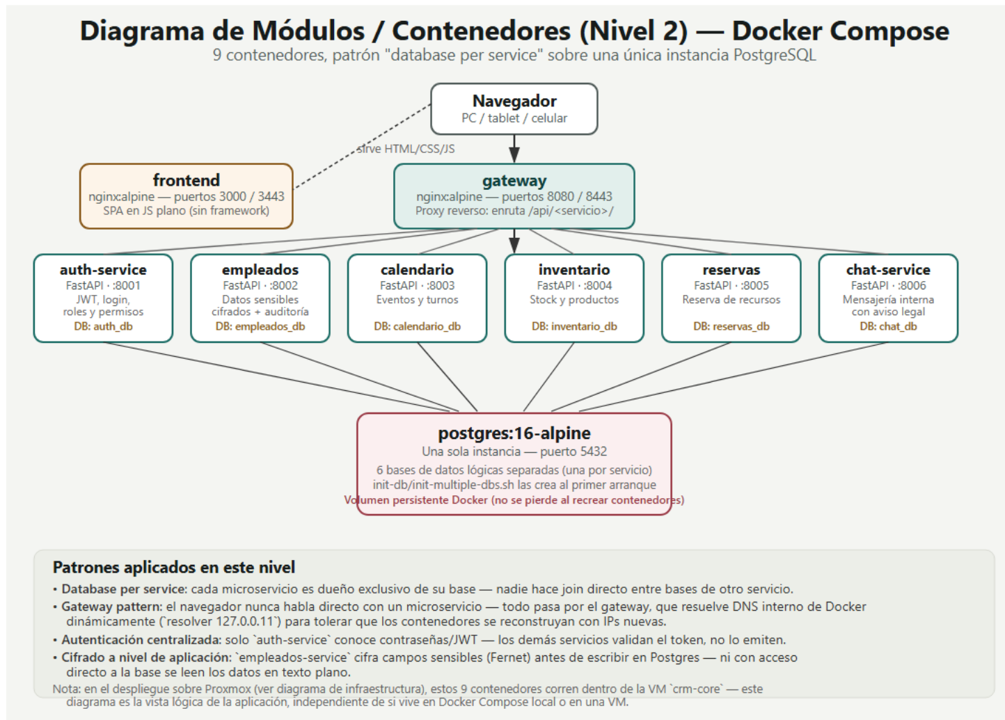
Figura 3. Diagrama de módulos / contenedores (nivel 2)
