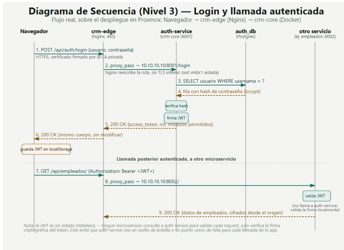
Figura 4. Diagrama de secuencia (nivel 3)
