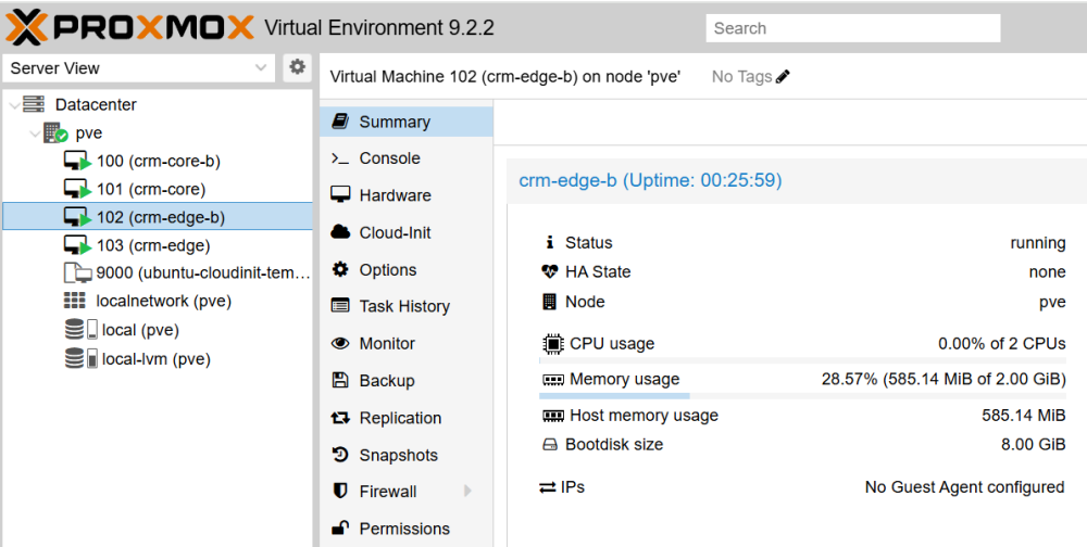
Figura 74. Resumen de crm-edge-b (VM 102)
