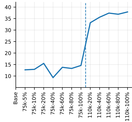
DS1000 Instruct
