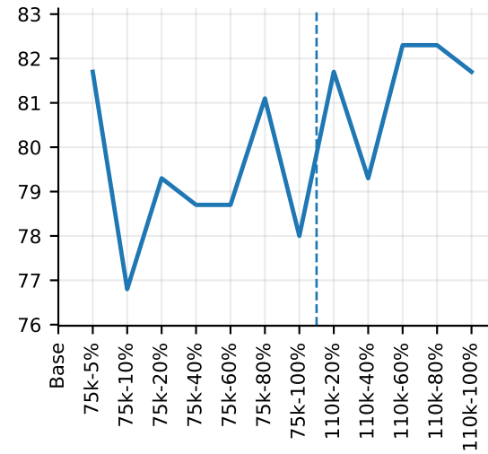
DS1000 Instruct
