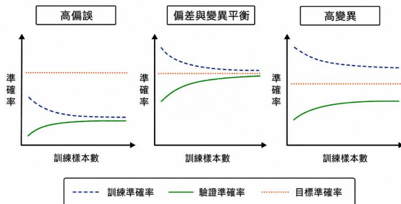
圖：三種學習曲線的類型
