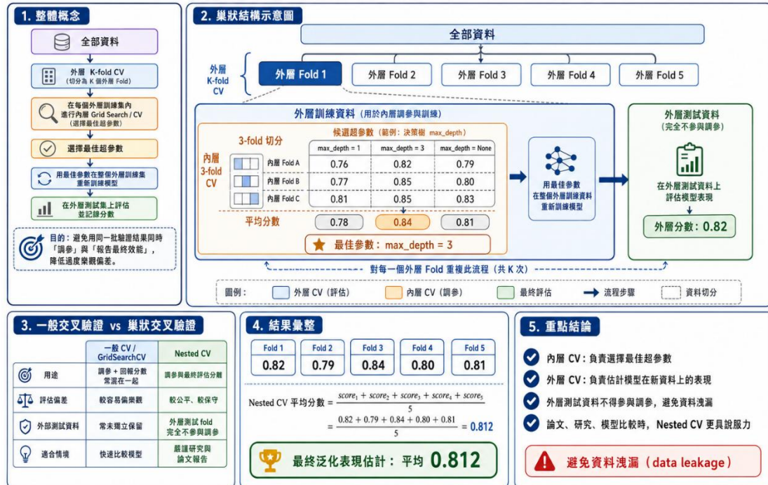
圖：巢狀交叉驗證的視覺化說明
