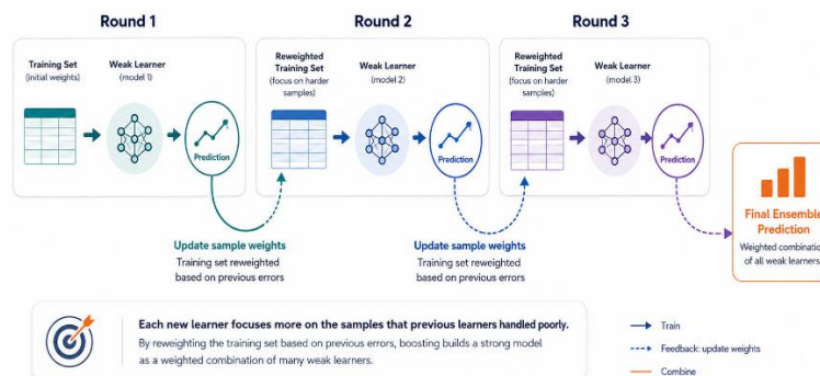
圖：提升法（Boosting）
