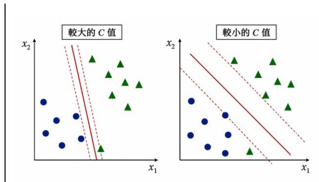
圖：不同超參數 C 值對 SVM 邊距的影響
