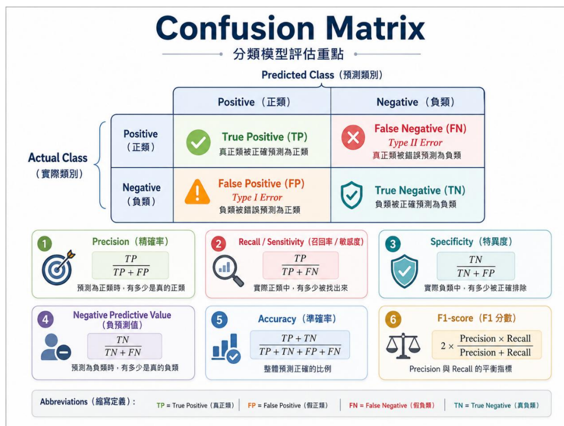
圖：用在二元分類的混淆矩陣
