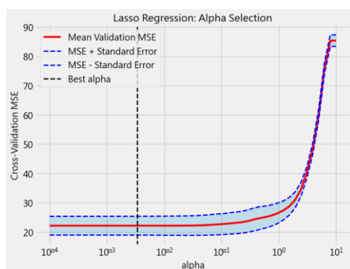
圖：用於 Lasso Regression 的 Alpha 選擇
