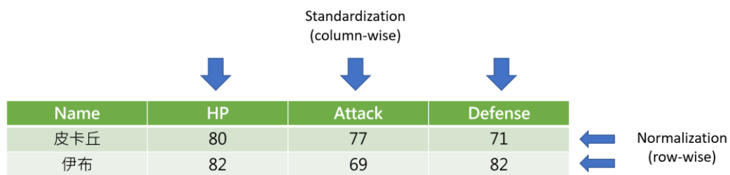
圖：對欄位進行標準化；對樣本進行正規化
