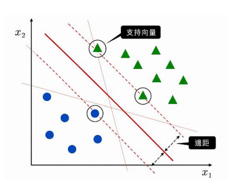
圖：支援向量機 SVM
