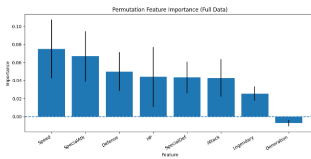
圖：不切分資料，直接列出特徵重要性
