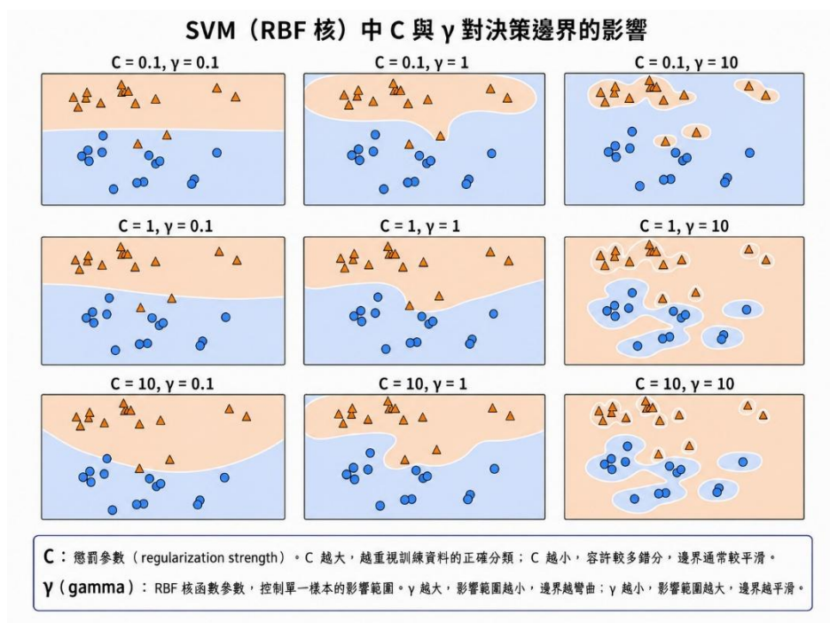
圖：使 kernel function 在不同 C 和 gamma 參數值的分類效果
