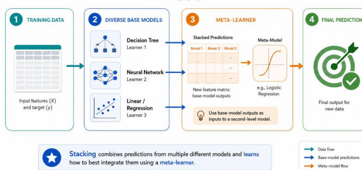
圖：堆疊法（Stacking）
