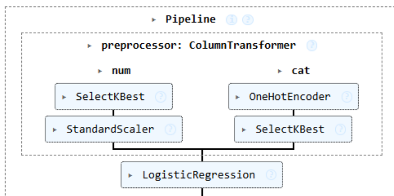
圖：完整的 Pipeline 圖形結構
