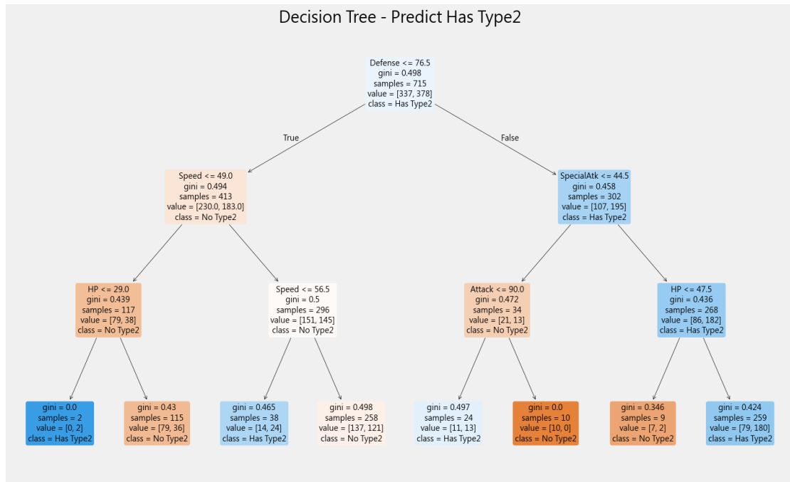
圖：決策樹的決策過程
