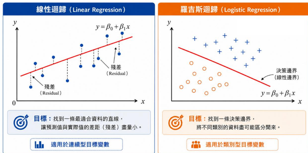
圖：線性迴歸與羅吉斯迴歸的差異
