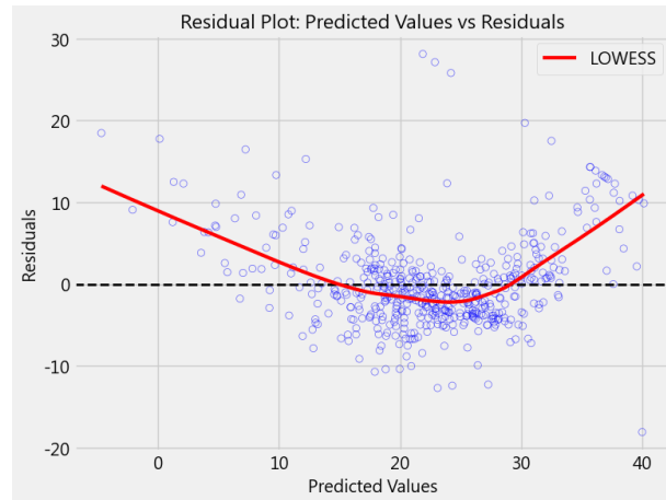
圖：模型可能沒有捕捉到非線性關係。
