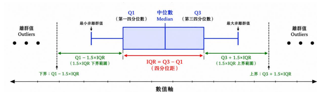
圖：IQR 圖解說明
