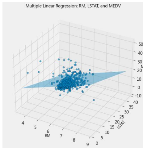
圖：3 維的多元線性迴歸視覺化
