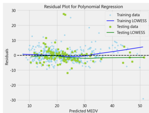
圖：多項式轉換後的特徵來進行殘差分析
