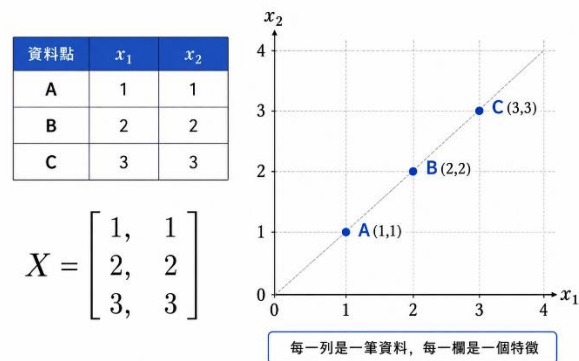
圖：原始的 2 維資料矩陣
