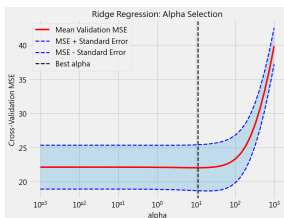
圖：用於 Ridge Regression 的 Alpha 選擇
