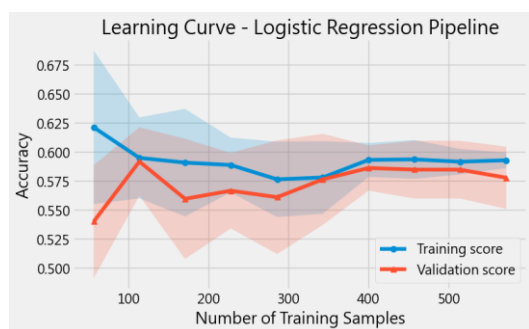
圖：兩個分數後期非常接近，沒有過擬合的問題，但兩者分數都不高，可能有欠擬合的問題。
