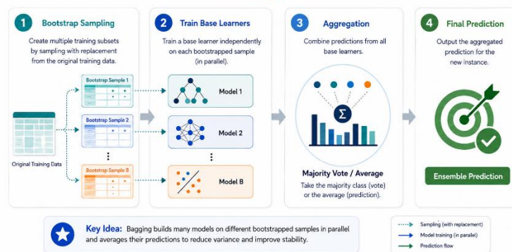
圖：袋裝法（Bagging）
