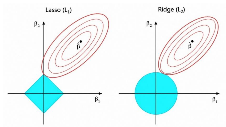
圖：Lasso 與 Ridge 的正規化效果
