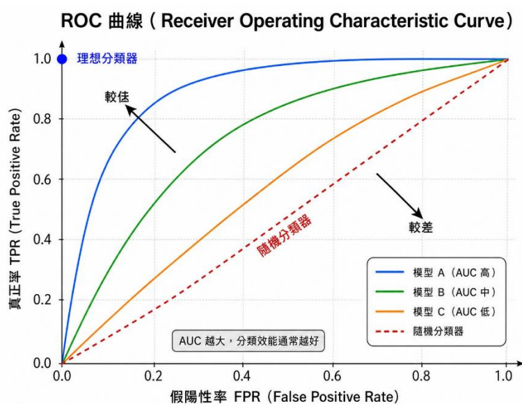
圖：ROC 曲線是用來觀察不同分類門檻下，TPR 與 FPR 之間的關係。
