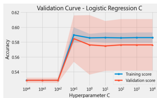
圖：當 C 繼續變大時，驗證分數沒有繼續提升，這代表讓模型更複雜，並沒有帶來更好的泛化能力。
