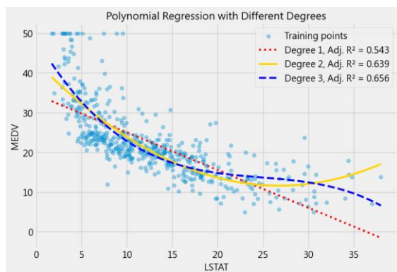
圖：不同次方用在多項式迴歸模型
