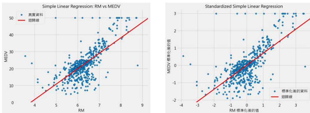
圖：檢視資料散佈程度與繪製迴歸線
