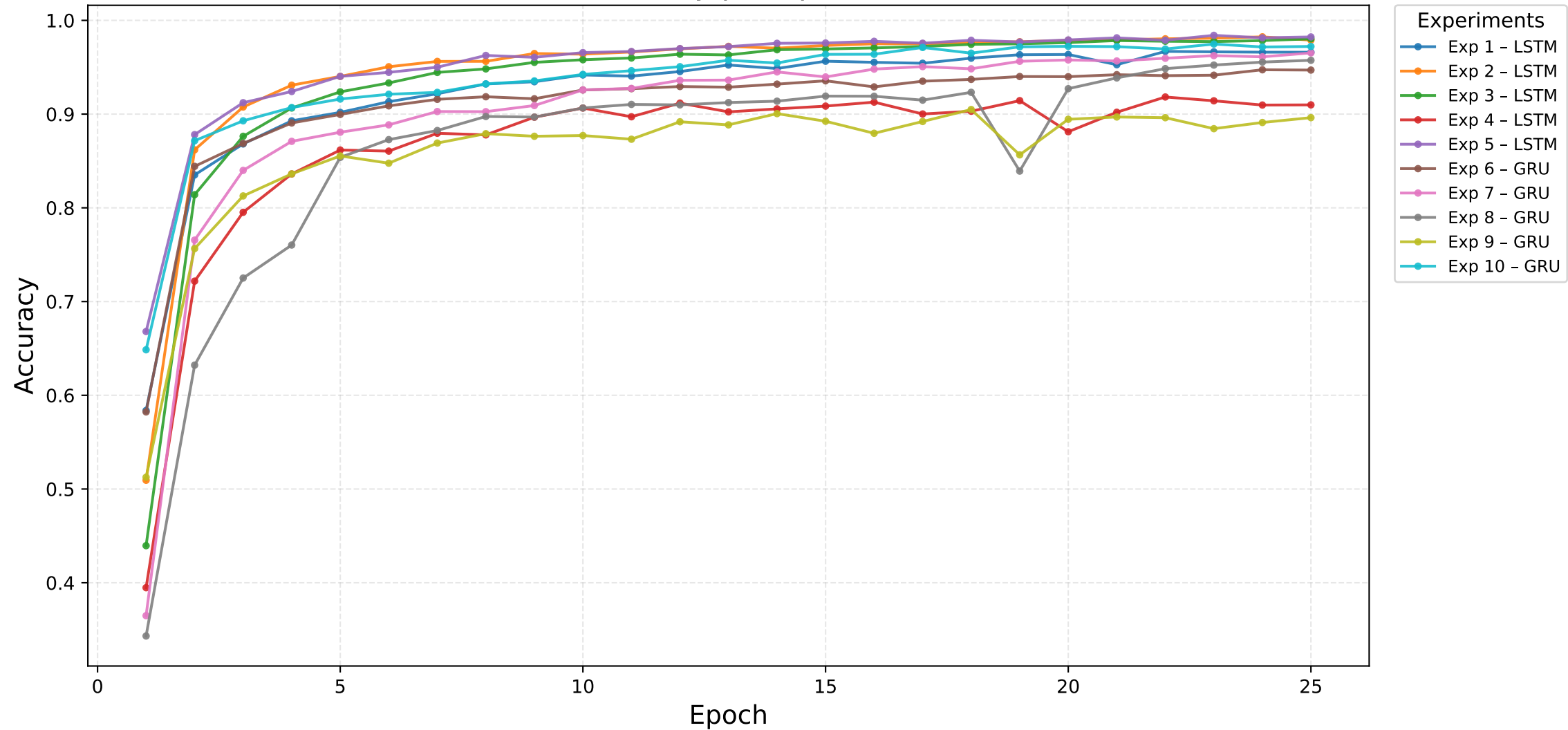
Accuracy per Epoch
