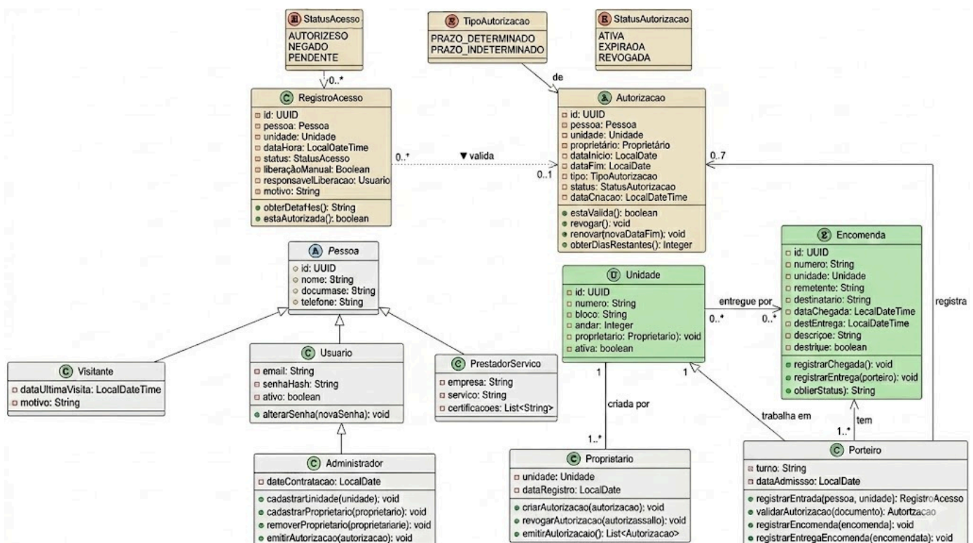
Figura 2: Diagrama de Classes demonstrando a aplicação de Herança e Associações.
