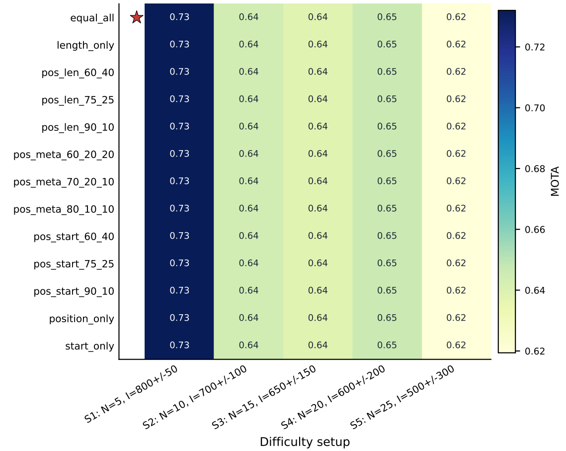
Trajectory-to-trajectory MOTA
