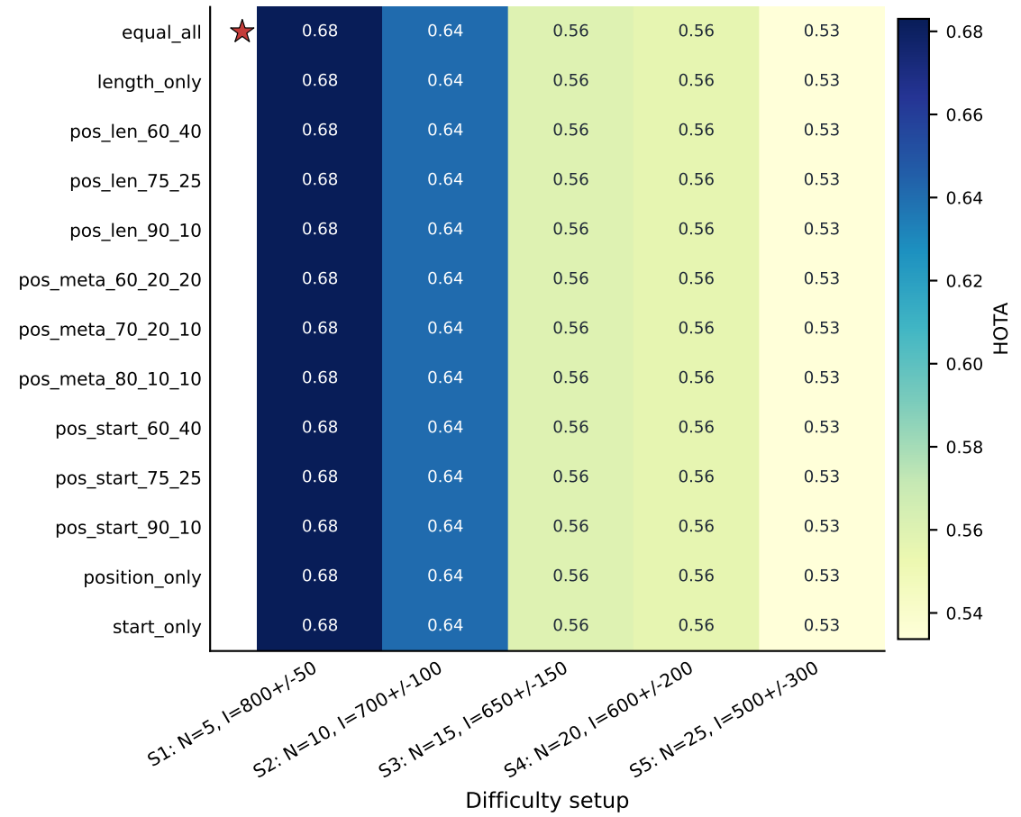
Trajectory-to-trajectory HOTA
