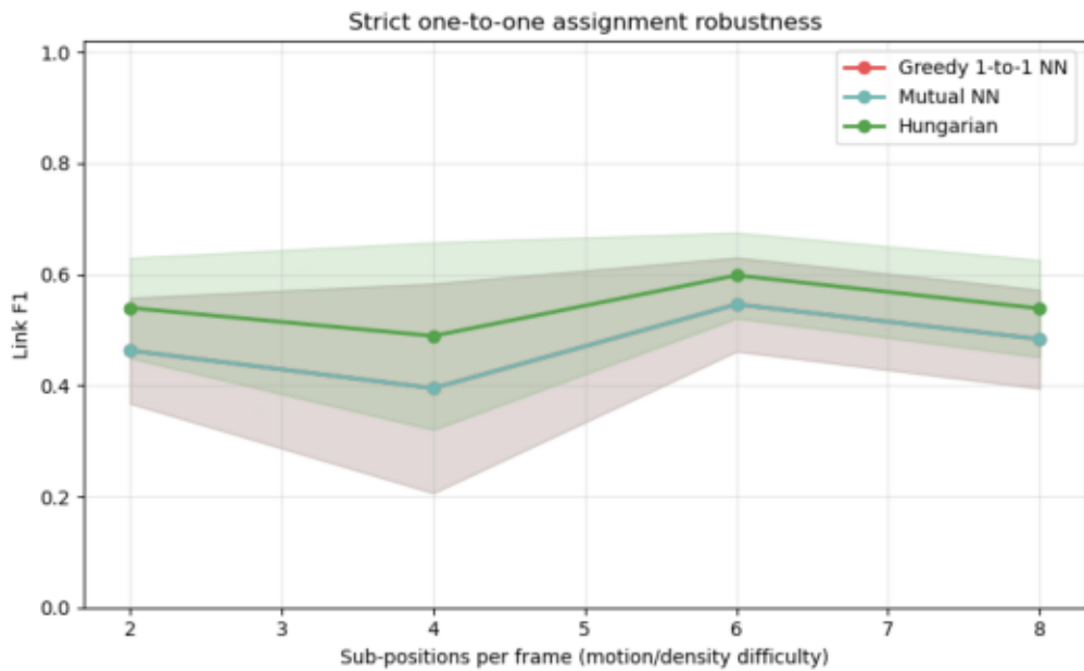
Strict 1-to-1 F1
