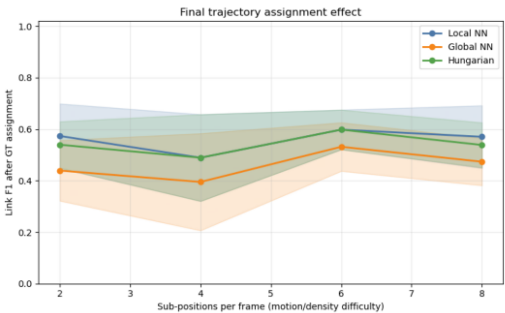
Trajectory assignment F1
