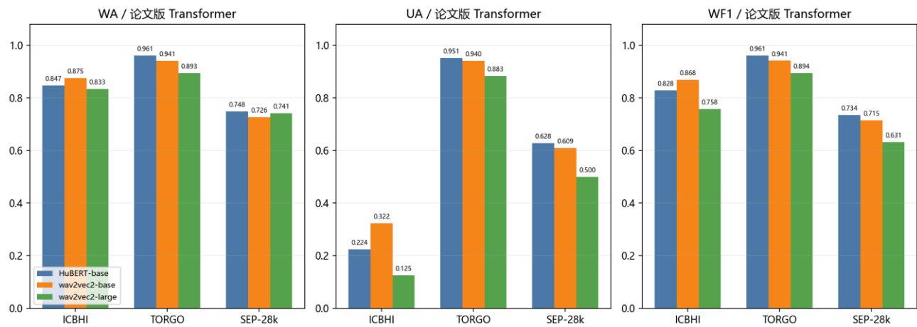
图 2 论文版 Transformer 在三个任务上的 WA、UA、WF1
