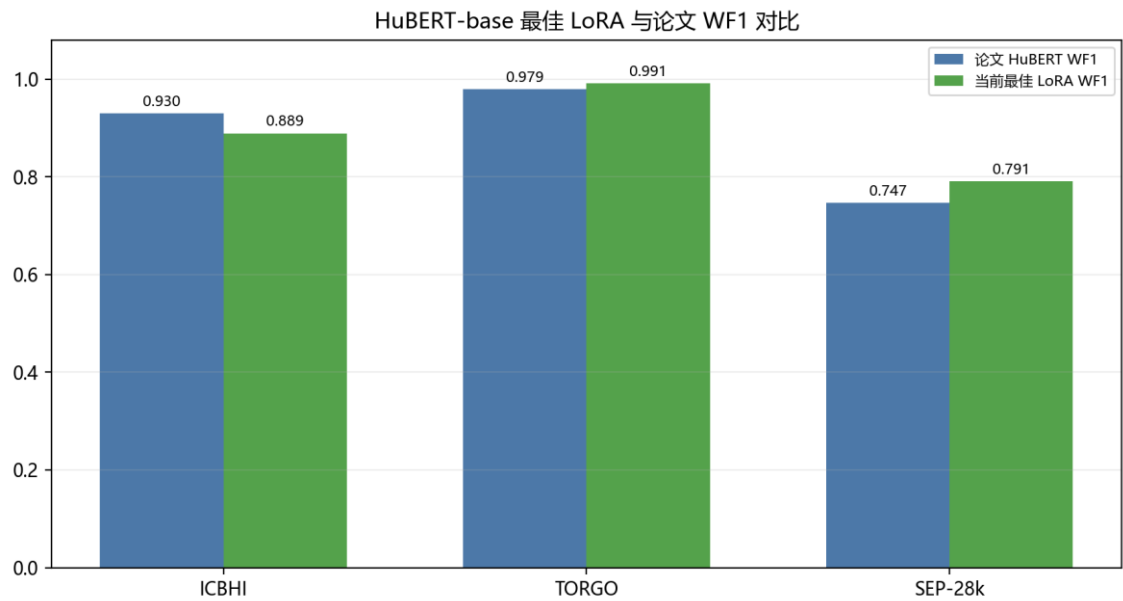
图 5 三个任务的最佳 LoRA WF1 与论文 HuBERT-base 对比
