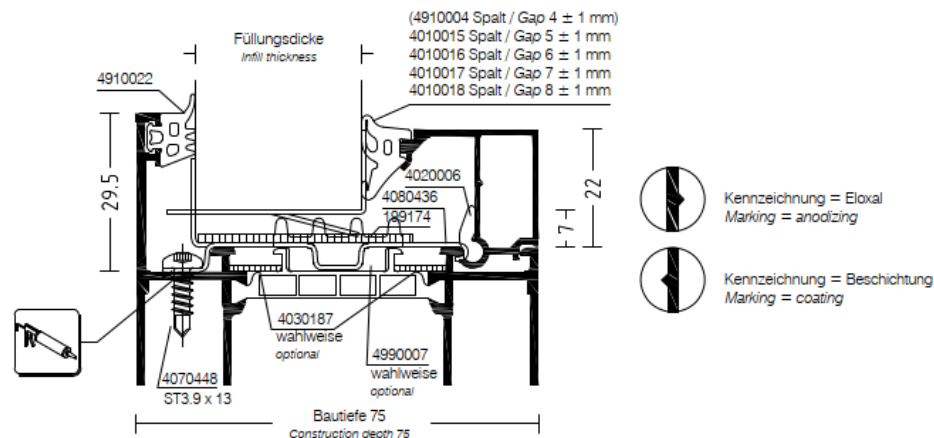
Bautiefe 75 - Verglasungsdichtung außen 4910022 Construction depth 75 mm - Outer glazing gasket 4910022
