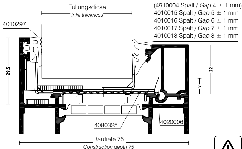
Bautiefe 75 - Verglasungsdichtung außen 4010297 Construction depth 75 mm - Outer glazing gasket 4010297
