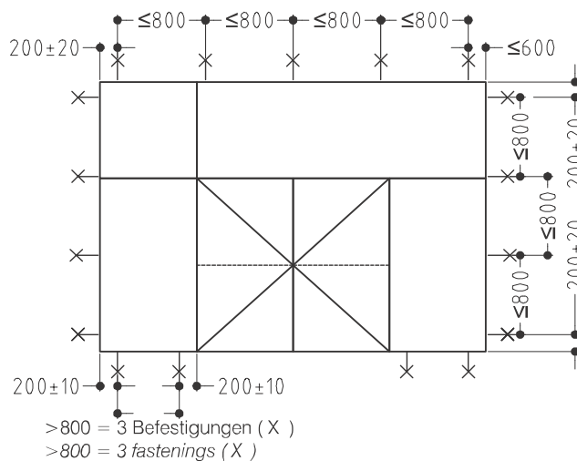
T-Bauteil Zweiflügelige Anschlagtür (in Vorbereitung) T-component Double leaf hinged door (in preparation)
