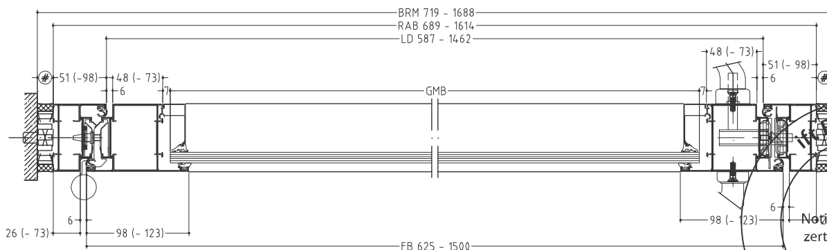
Grundvariante Basic variant
