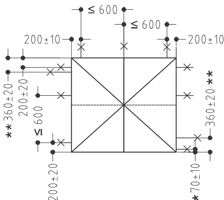
Zweiflügelige Anschlagtür Double leaf hinged door
