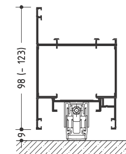
Flügelprofile Sash profiles
