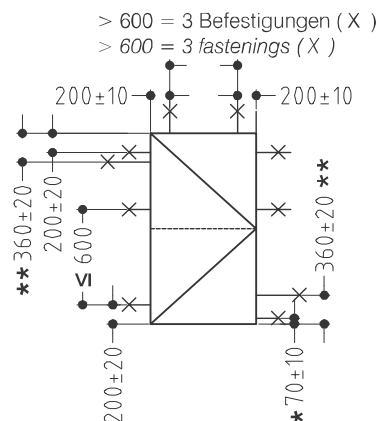
Einflügelige Anschlagtür Single leaf hinged door
