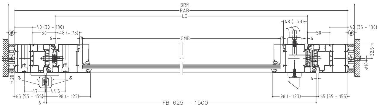
Grundvariante Basic variant
