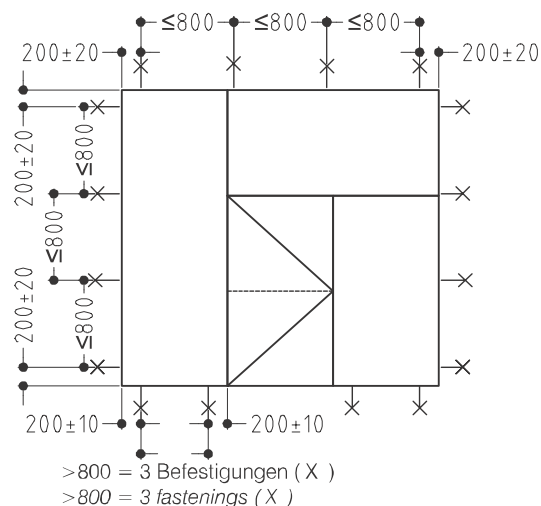
T-Bauteil Einflügelige Anschlagtür (in Vorbereitung) T-component Single leaf hinged door (in preparation)
