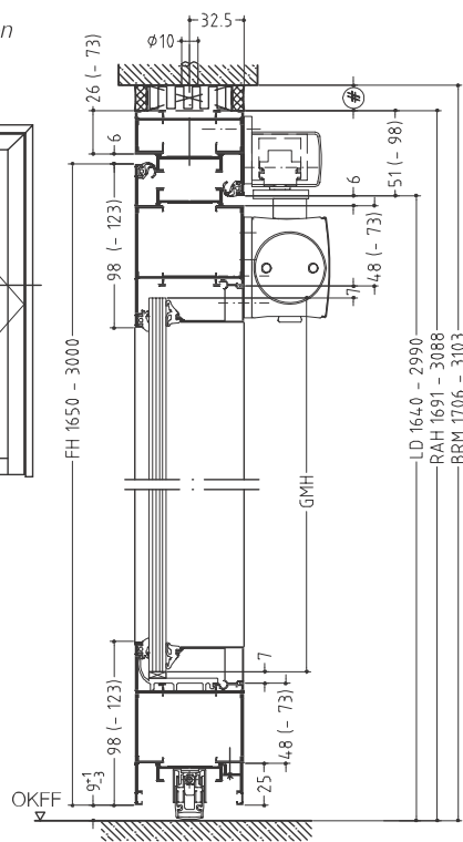
Grundvariante Basic variant
