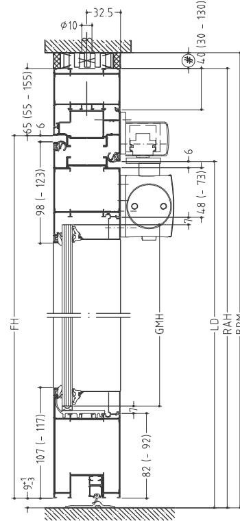
Blendrahmenvariante Frame variant
