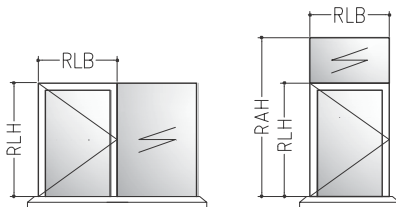
Tür und Festfelder mit Verglasungen Door and fixed fields with glazings
