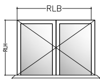
EW30 - C 5 S 200 Zweiflügelige Anschlagtür Double leaf hinged door
