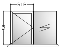
EW30 - C 5 S 200 Tür EW30 - C 5 S 200 Door
