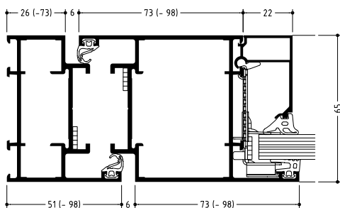
WICSTYLE 65N NG FP Brandschutztür EW 30
