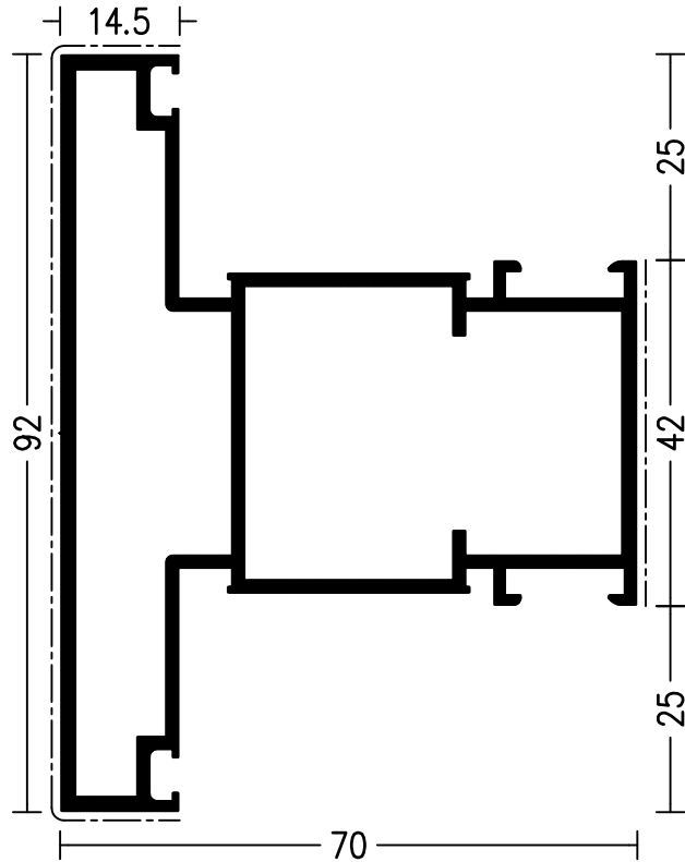
132346 Kämpferprofil
