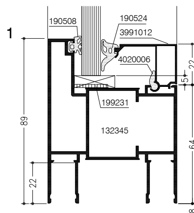
Blendrahmen als Sockelprofil
