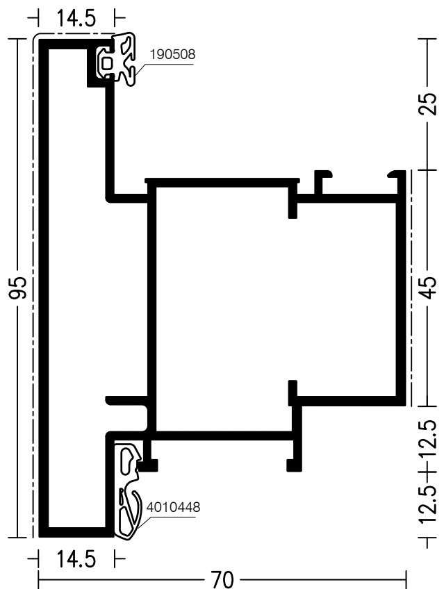
132343 Anschlagtür auswärts
