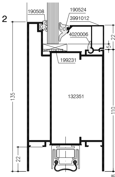
Anschlagtür nach außen öffnend mit Oberlicht
