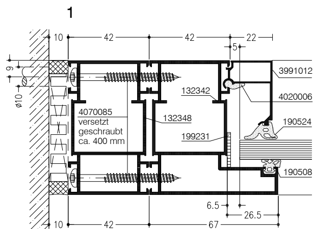
Blendrahmen-Verbreiterungsprofil
