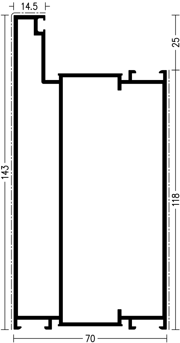
132352 Sockelprofil für Festfeld
