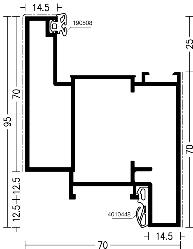
132344 Anschlagtür einwärts
