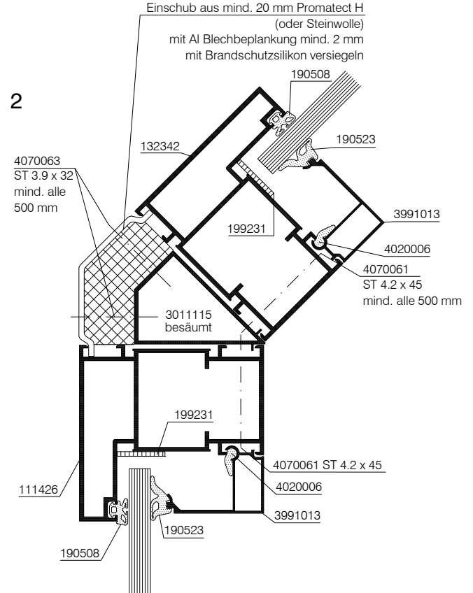
45° Knick horizontal
