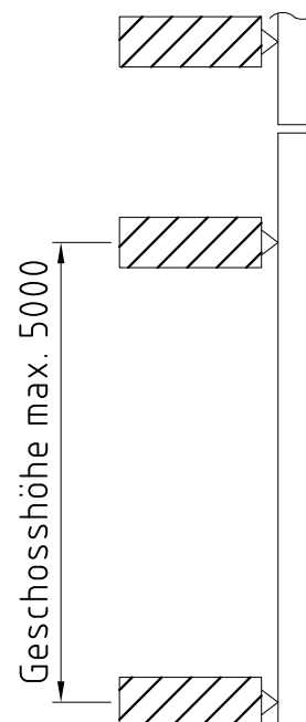
Vorgehängte Fassade
