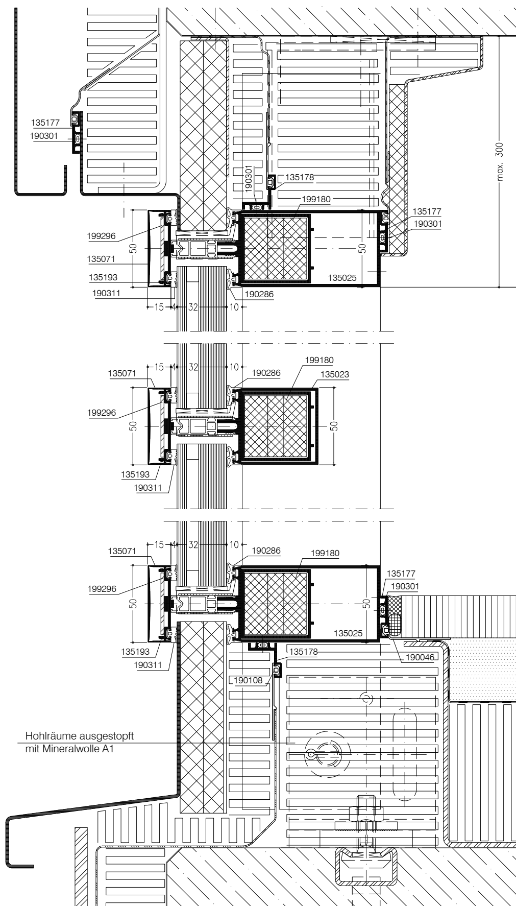
Vertikalschnitt, F50FPA001
