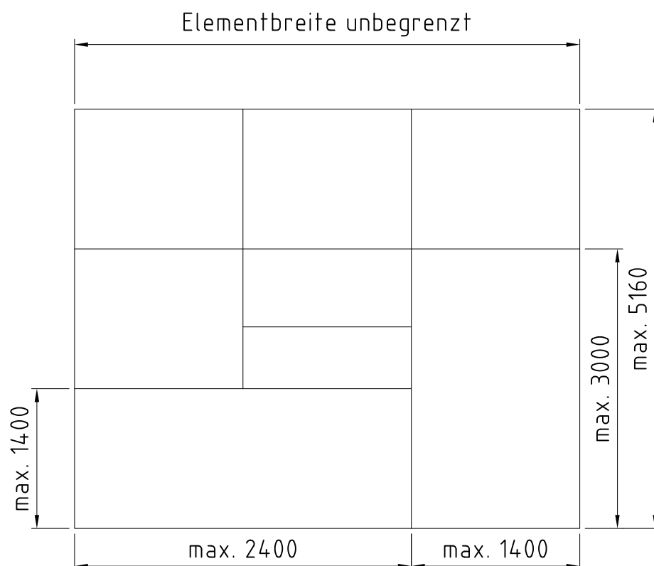
Eingestelle Fassade
