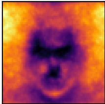
Layer 2
