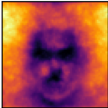
Layer 3
