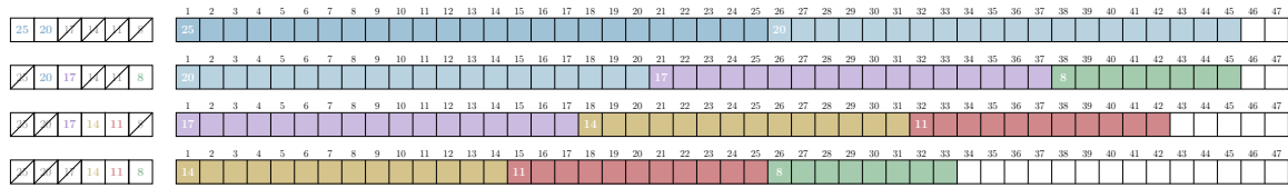
FIGURE 9 – Application de l'algorithme glouton répété sur l'instance #21 : S_1 = \{14, 11, 8\} .
