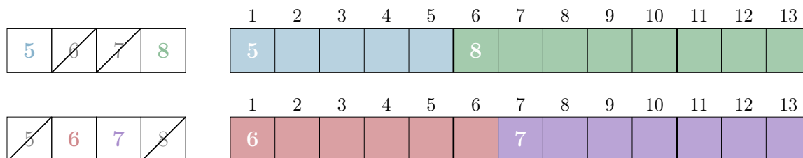
FIGURE 2 – Partition parfaite de quatre entiers consécutifs.
