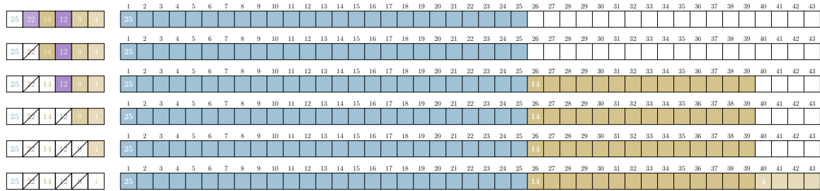
FIGURE 5 – Application de l'algorithme glouton sur l'instance #1 : S_1 = \{25, 14, 4\} .
