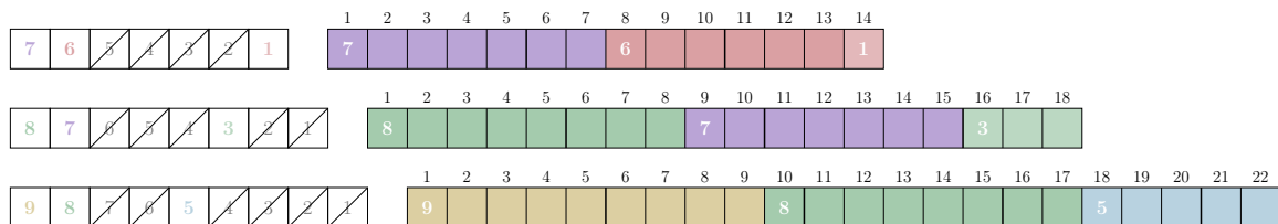
FIGURE 4 – Partition parfaite des entiers de 1 à n pour n = 7, 8, 9 .
