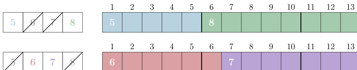
FIGURE 2 – Partition parfaite de quatre entiers consécutifs.
