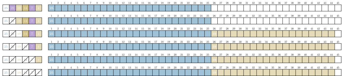
FIGURE 6 – Application de l'algorithme glouton sur l'instance #11 : S_1 = \{25, 19\} .
