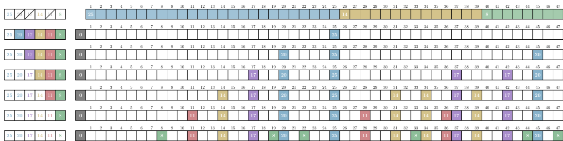
FIGURE 10 – Application de la programmation dynamique sur l’instance #21 : S_1 = \{25, 14, 8\} .
