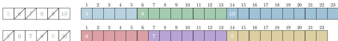
FIGURE 3 – Partition parfaite de six entiers consécutifs.
