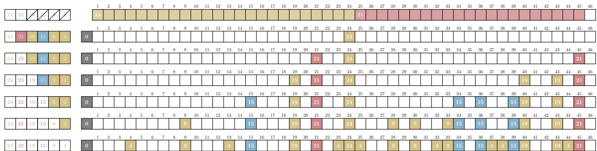
FIGURE 10 – Application de la programmation dynamique sur l'instance #31 : S_1 = \{24, 21\} .
