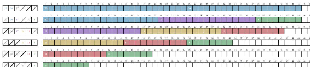
FIGURE 5 – Application de l’algorithme glouton répété sur l’instance #13.
