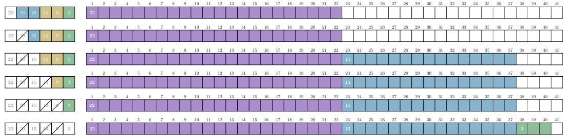
FIGURE 2 – Application de l’algorithme glouton sur l’instance #7.
