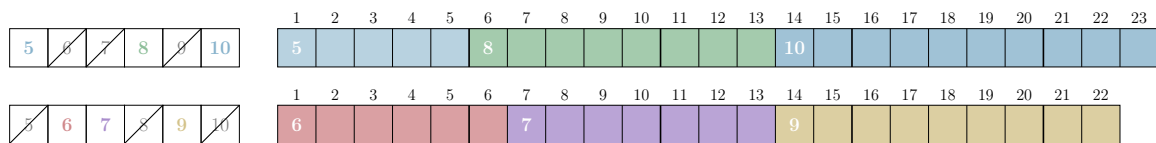
FIGURE 3 – Partition parfaite de six entiers consécutifs.
