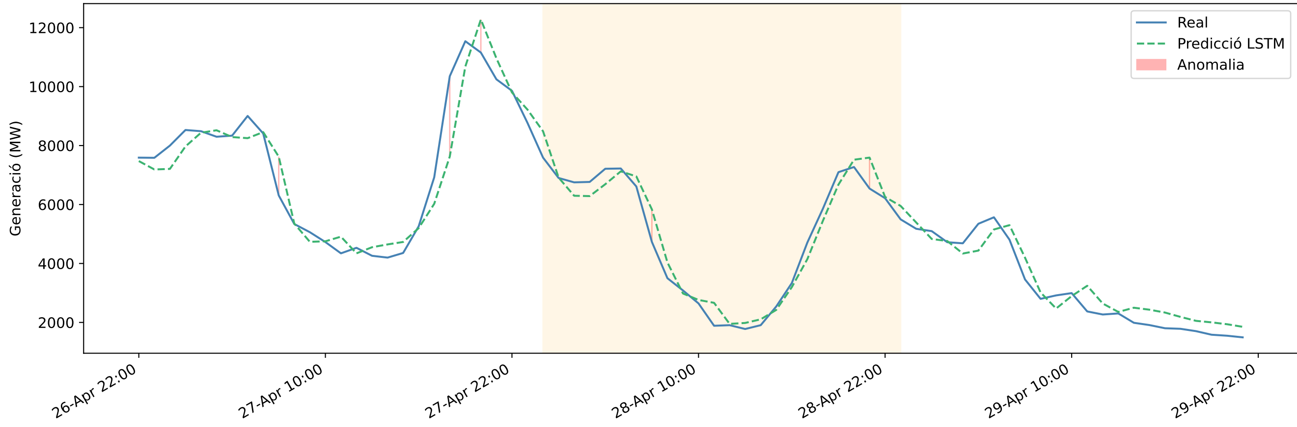
LSTM - Eòlica | Detall apagada 27-29 abril 2025
