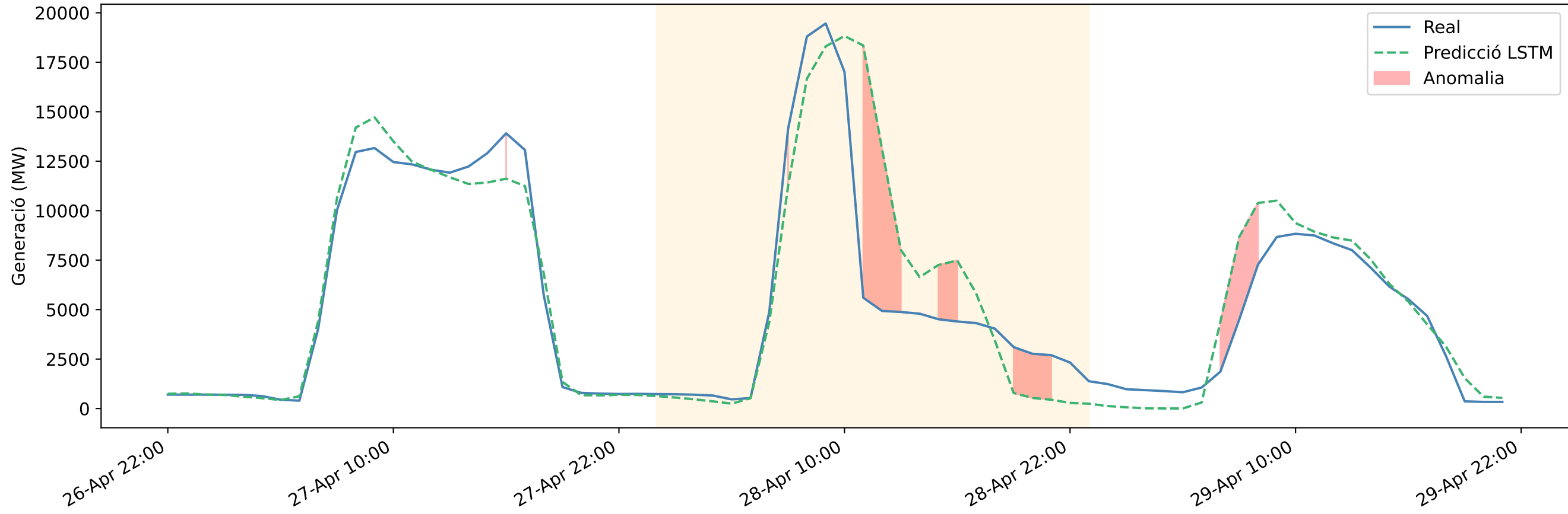
LSTM - Solar PV | Detall apagada 27-29 abril 2025
